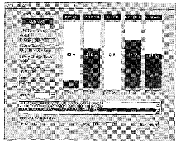
그림 4 접속 화면 (LINE: UPS 입력 저전압) Fig. 4 Connected UPSMonitor (LINE: UPS Input Low Voltage)
