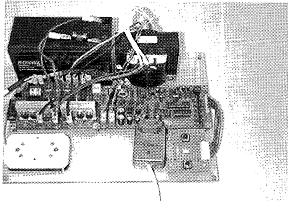
그림 1 1KVA UPS Proto Type Fig. 1 1KVA UPS Proto Type
