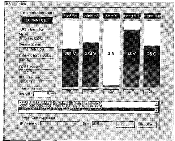
그림 3 접속 화면 (LINE: Step-Up) Fig. 3 Connected UPSMonitor (LINE: Step-Up)
