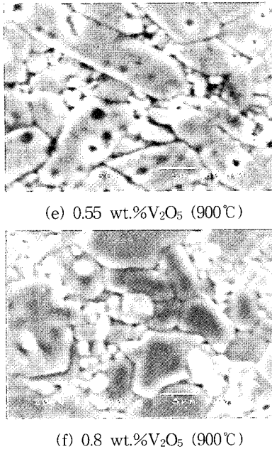
그림 3. 870°C와 900°C에서 5시간 소결한 (Zn_{0.8}Mg_{0.2})TiO_3 + (1-x) wt.\%Bi_2O_3 + x wt.\%V_2O_5 계의 Bi_2O_3 와 V_2O_5 첨가량에 따른 주사전자 현미경 미세구조. (a) x=0.2 wt.\% (b) x=0.55 wt.\% (c) x=0.8 wt.\% (870°C/5h) ; (d) x=0.2 wt.\% (e) x=0.55 wt.\% (f) x=0.8 wt.\% (900°C/5h).
