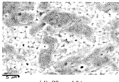
(d) 20 mol.%
