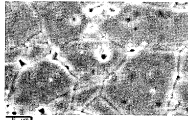
(b) 9 mol.%
