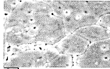
(a) 5 mol.%
