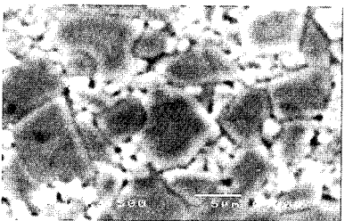
(d) 0.2 wt.%V 2 O 5 (900°C)
