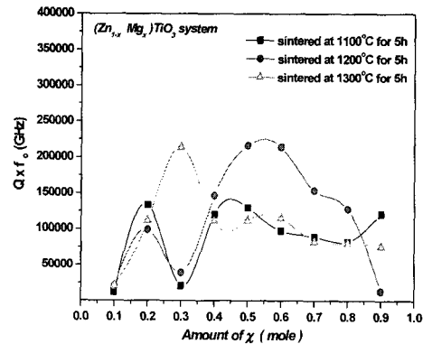
그림 1. 1100°C~1300°C에서 5시간 소결한 (Zn_{1-x}Mg_x)TiO_3 계의 Q \times f_0 (GHz)값의 변화.
