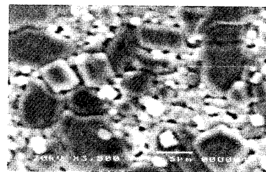
(a) 0.2 wt.%V 2 O 5 (870°C)
