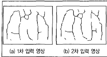
그림 7 세션화 영상
