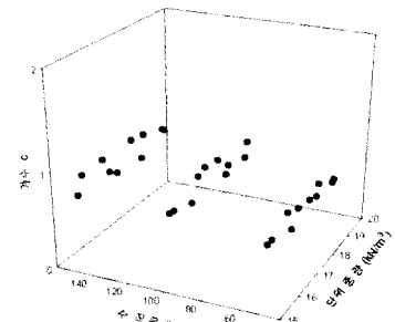
(c) 계수 c 의 경향
