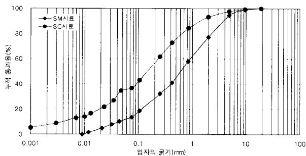
그림 4. 시험시료 입도분포곡선
