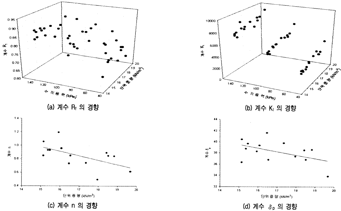
그림 8. SM토질에서의 쌍곡선 모델 계수 경향
