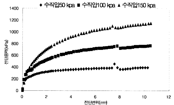
그림 5. 전단변형-응력 관계곡선
