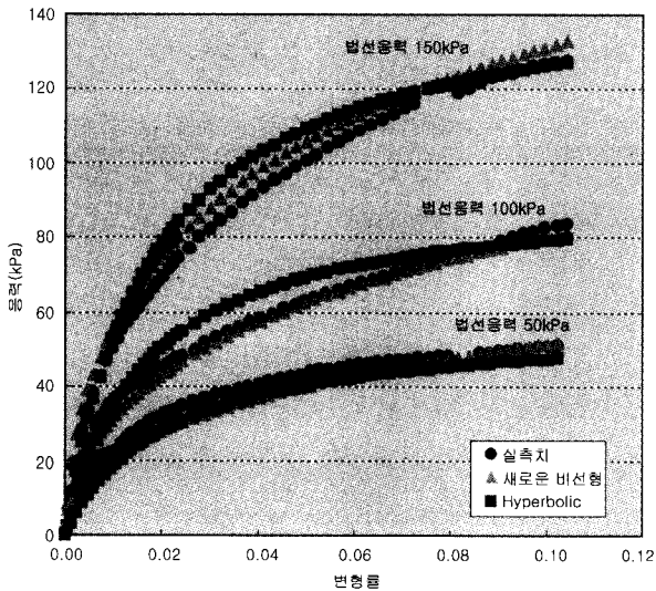
그림 13. 단위중량 17.96 kN/m 3 , SM 토질의 실측치와 예측모델들과의 비교
