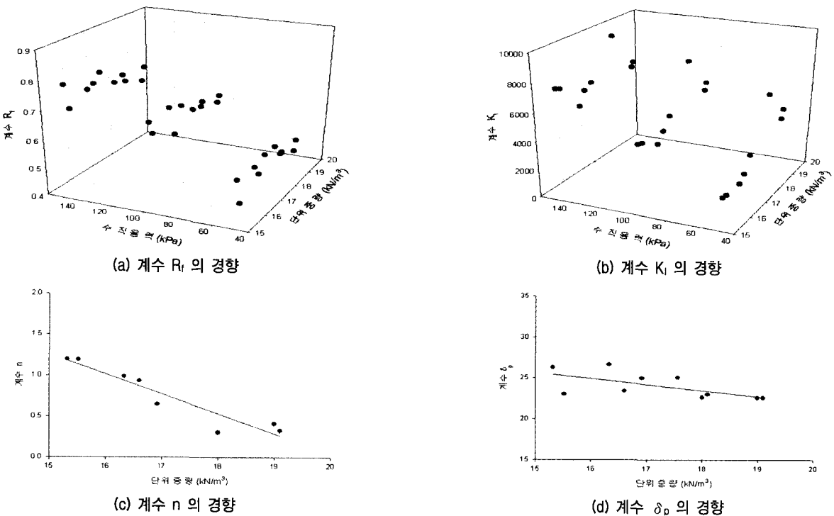
그림 9. SC토질에서의 쌍곡선 모델 계수 경향
