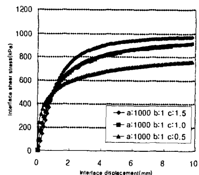
(c) 계수 c의 특성
