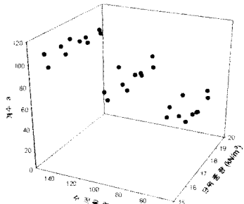
(a) 계수 a 의 경향
