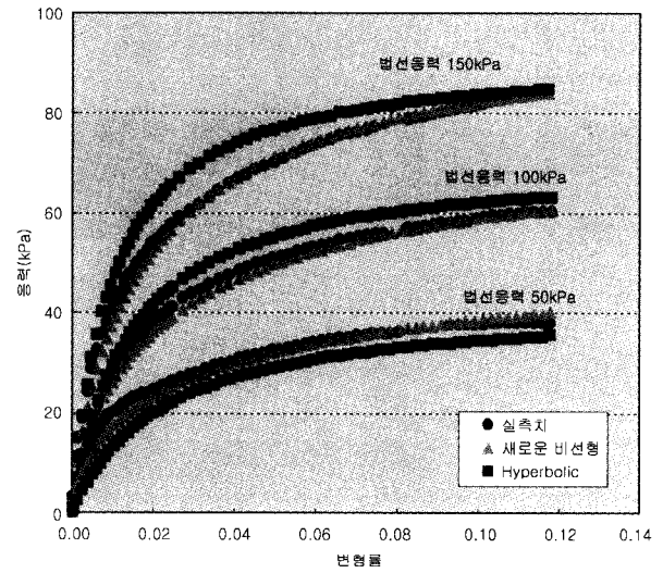
그림 14. 단위중량 16.92 kN/m 3 , SC 토질의 실측치와 예측모델들과의 비교
