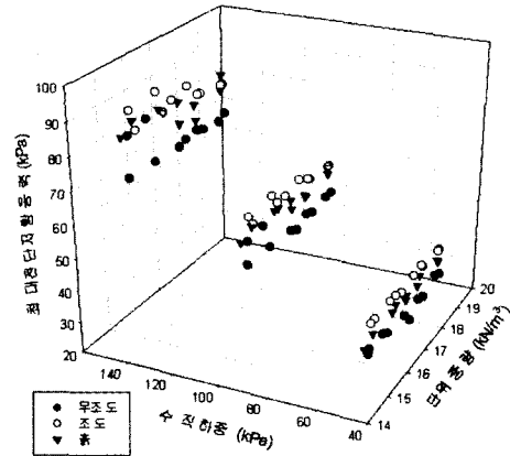
그림 7. 최대 주면전단 저항응력(SM시료)
