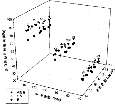
그림 6. 최대 주면전단 저항응력(SC시료)
