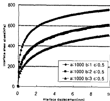
(b) 계수 b의 특성
