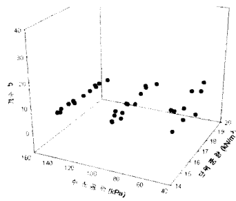
(b) 계수 b 의 경향
