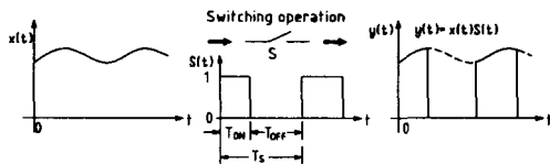
그림 5. 입출력 전압과 존재함수 Fig. 5. Input and output voltage and existence function
