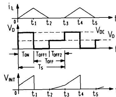
그림 8. 전류 불연속 모드에서 주요 동작 파형 Fig. 8. Operation waveform
