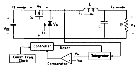
그림 2. 강압형 DC-DC 컨버터의 순시추종 PWM 제어 Fig. 2. Instantaneous following PWM control of buck converter
