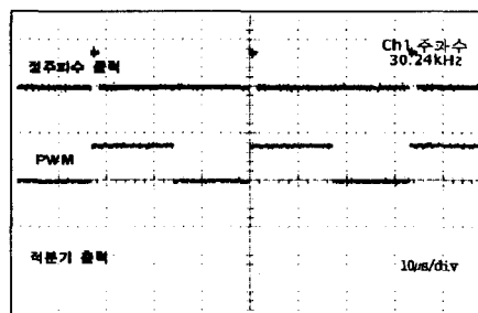
(b) 제어회로의 실측 파형
