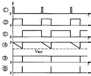
(a) 제어회로의 주요 파형
