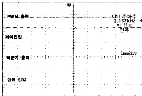
그림 11. 제어 기준값이 변할 때 제어기의 추종 특성 Fig. 11. Following characteristics of controller when the reference voltage fluctuate
