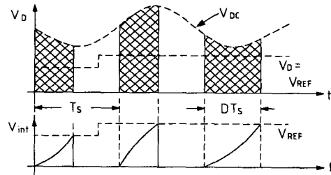
그림 4. 전원전압이 변동될 때 기준전압 가변제어 Fig. 4. Reference voltage variable control when the source voltage fluctuate
