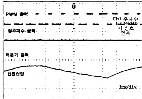
그림 10. 전원 전압이 변동될 때 제어기의 보상 특성 Fig. 10. Compensation characteristics of controller when the source voltage fluctuate
