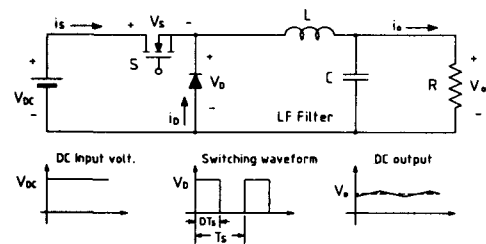
그림 1. 강압형 DC-DC 컨버터 회로와 동작파형 Fig. 1. Circuit and operation waveform of buck converter
