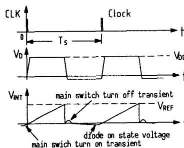
그림 9. 스위칭 소자의 스위칭 특성과 적분전압 Fig. 9. Integral voltage and switching characteristics of device
