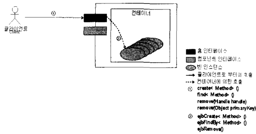
그림 5 Persistence CRUD(PC) 패턴
