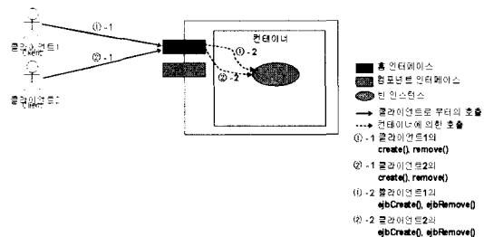
그림 13 Common Instance CRUD(CIC) 패턴
