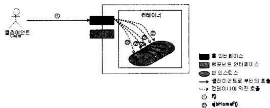
그림 3 Static Business(SB) 패턴
