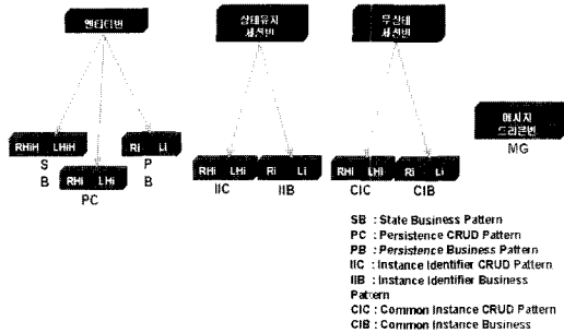
그림 20 각 인터페이스별 패턴 적용 유형
