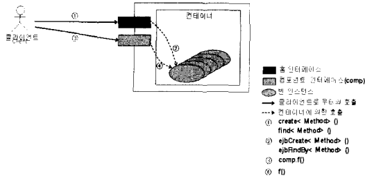
그림 7 Persistence Business(PB) 패턴
