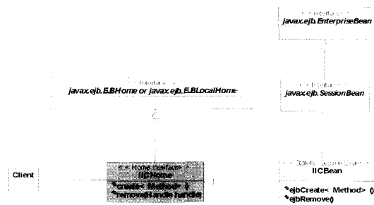
그림 10 상태유지 세션 빈의 홈 인터페이스 관련 클래스 구조
