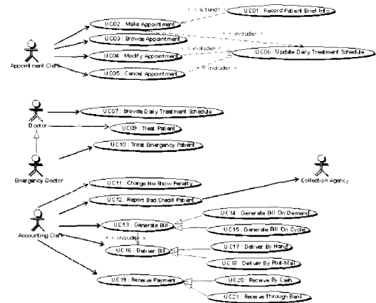
그림 21 병원 관리 시스템의 Use Case 다이어그램
