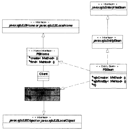
그림 8 엔티티 빈의 컴포넌트 인터페이스 관련 클래스 구조
