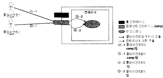
그림 15 Common Instance Business(CIB) 패턴
