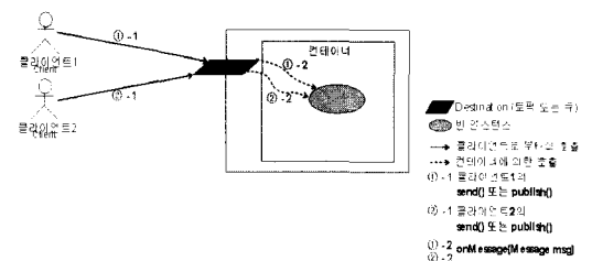
그림 17 Message Grasp(MG) 패턴
