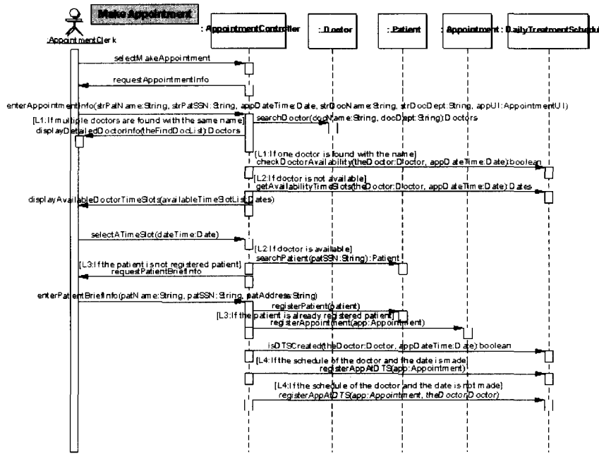
그림 24 병원 관리 시스템의 시퀀스 다이어그램 1
