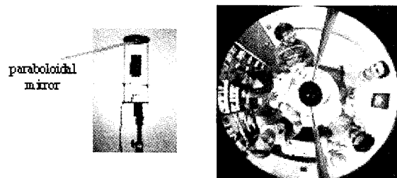
(그림 1) 전방향성 카메라 (a) 전방향성 카메라 (b) 획득된 영상
