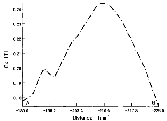
그림 6 고압 권선에서의 수직자장의 분포 Fig. 6 Distribution of perpendicular B on the high voltage winding
