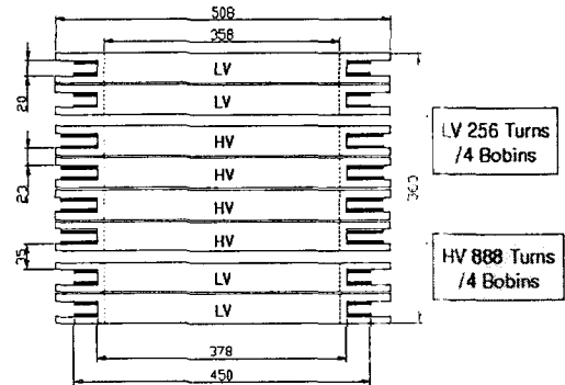
그림 2 더블 팬케이크 권선의 치수와 배열 Fig. 2 Dimension and arrangement of the double pancake windings
