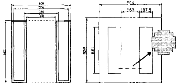
그림 3 냉동조와 외철형 철심의 치수 Fig. 3 Dimension of the cryostat and the shell type core
