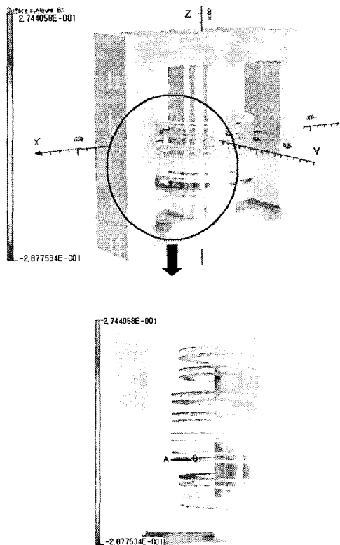
그림 5 1MVA 고온 초전도 변압기 권선에서의 B x 분포 Fig. 5 B x distribution of 1MVA HTS transformer
