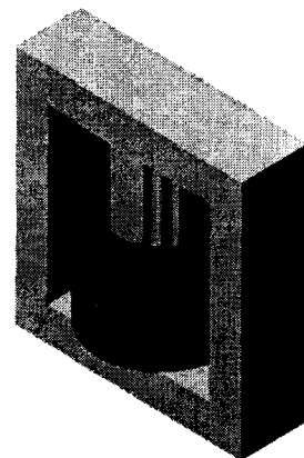
그림 4 1MVA 고온 초전도 변압기의 권선 드립 모델 Fig. 4 Total arrangement of the 1MVA HTS transformer
