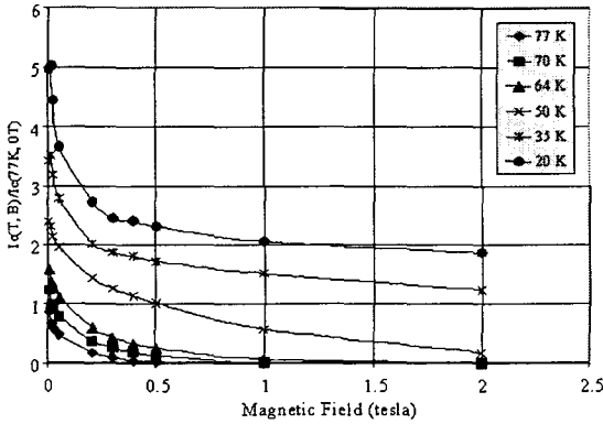
그림 1 온도에 따른 선재 표면에 수직한 자장과 임계전류와의 관계 Fig. 1 Scaling ratios for temperature and magnetic field perpendicular to tape surface
