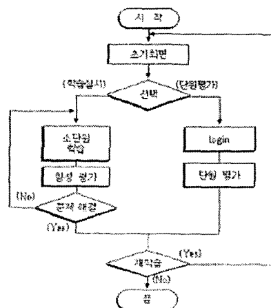
(그림 1) 학습 설계 흐름도
