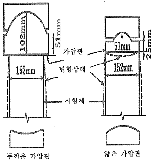
(그림 9) 시험체단부의 응력변형에 미치는 가압판의 영향
