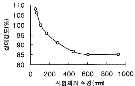
[그림 2] 압축강도시험결과에 미치는 시험체의 크기영향
