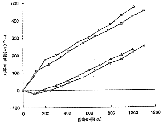
[그림 12] 재하시 나타나는 지주의 변형
