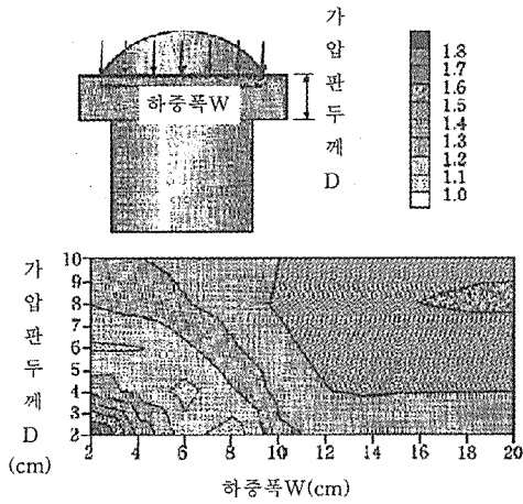
(그림 10) 구좌 · 가압판 변형 · 크기와 시험체상부 최대압축응력과의 관계
