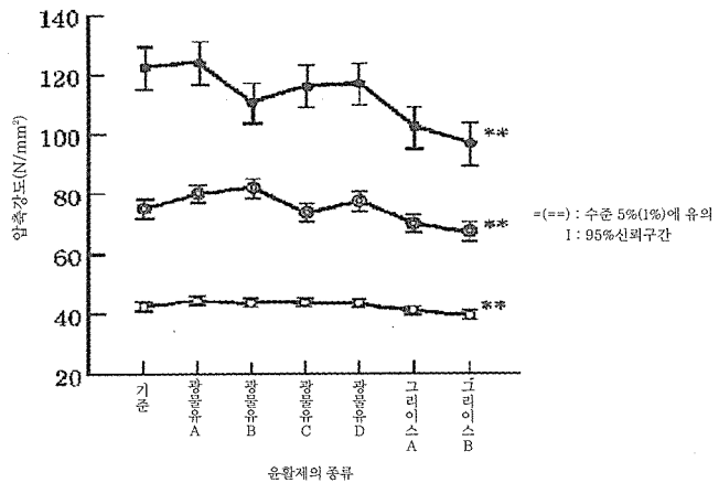
(그림 11) 압축강도시험결과에 미치는 구좌윤활제 종류의 영향
