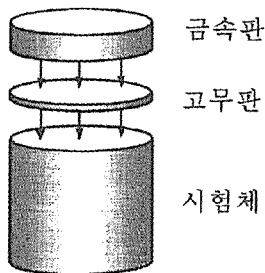
(그림 5) Unbonded Capping
