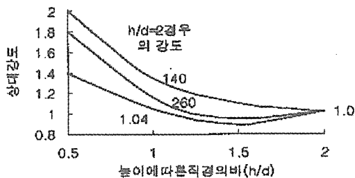
(그림 3) 압축강도시험결과에 미치는 높이와 직경의비 영향
