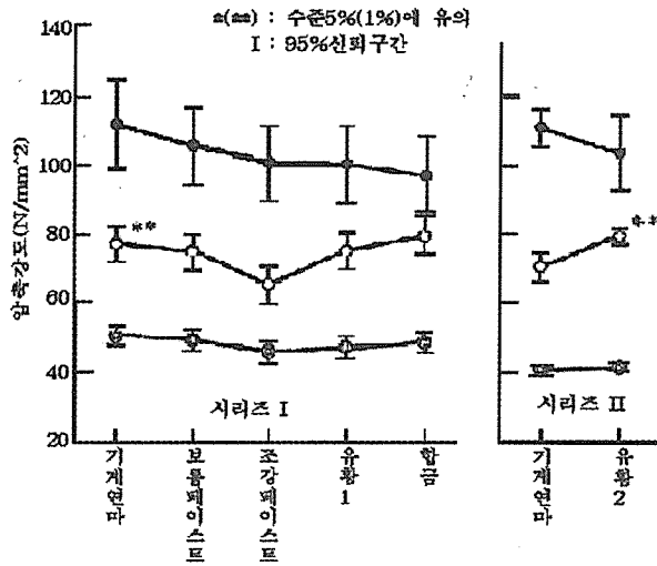
(그림 4) 압축강도시험결과에 미치는 단면처리 영향
