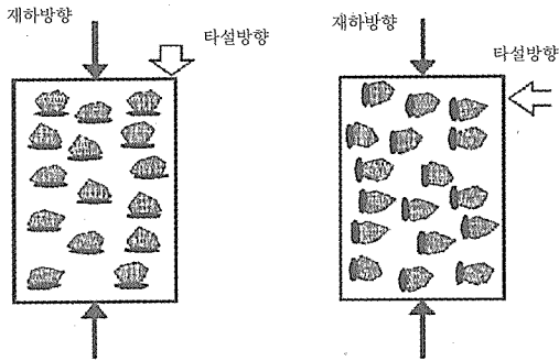
(그림 8) 콘크리트 타설방향과 재하방향의 관계
