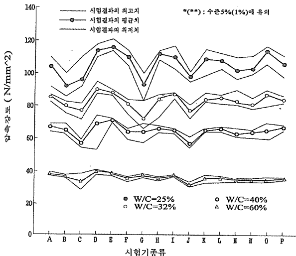
(그림 1) 압축강도시험결과에 미치는 시험기종류의 영향
