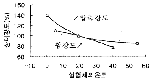
(그림 7) 압축강도시험결과에 미치는 시험체온도의 영향
