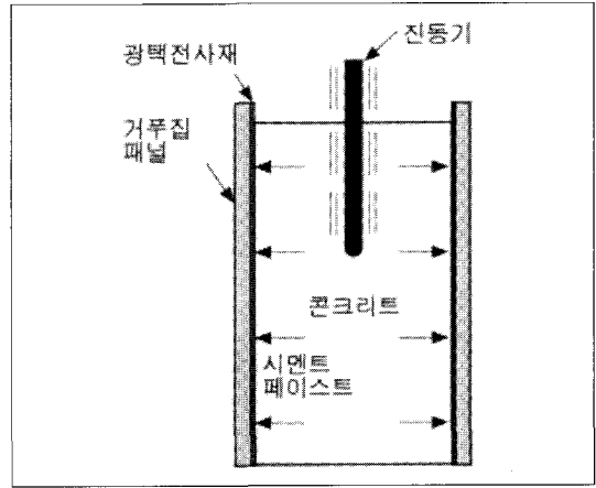
〈그림-2〉 거푸집면으로의 시멘트페이스트의 이동
