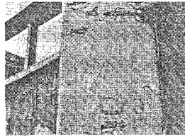
피복두께 부족에 의한 박리
