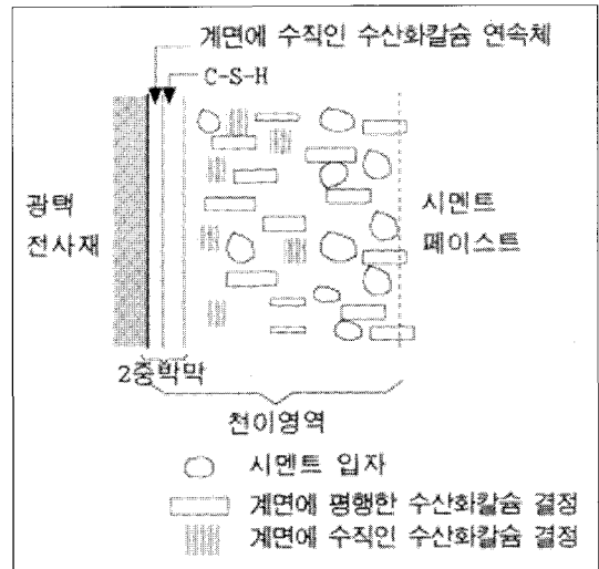
〈그림-3〉 천이영역 모델
