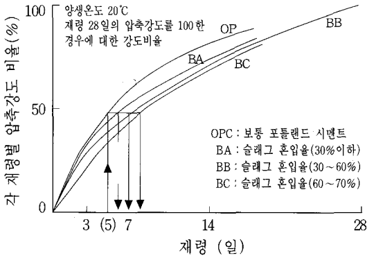
〈그림-3〉 시멘트 종류별 초기재령에서의 강도특성
