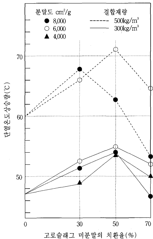
〈그림-2〉 콘크리트의 수화열과 치환율과의 관계
