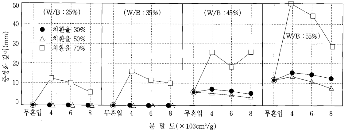
〈그림-5〉 촉진 중성화시험에 의한 시험결과(촉진 1개월)
