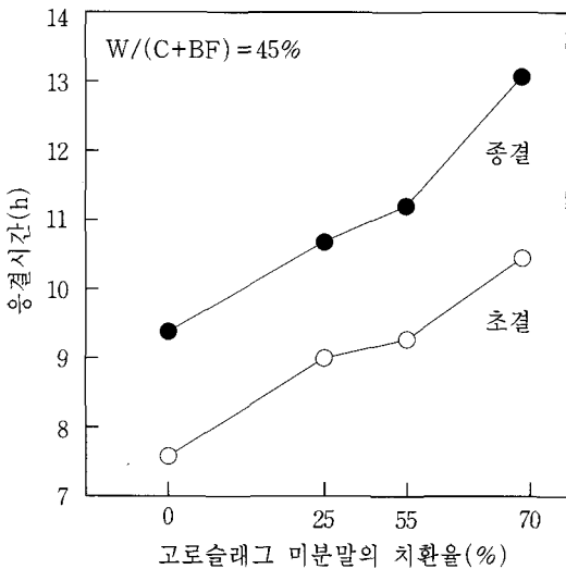
〈그림-1〉 슬래그의 치환율과 응결시간과의 관계
