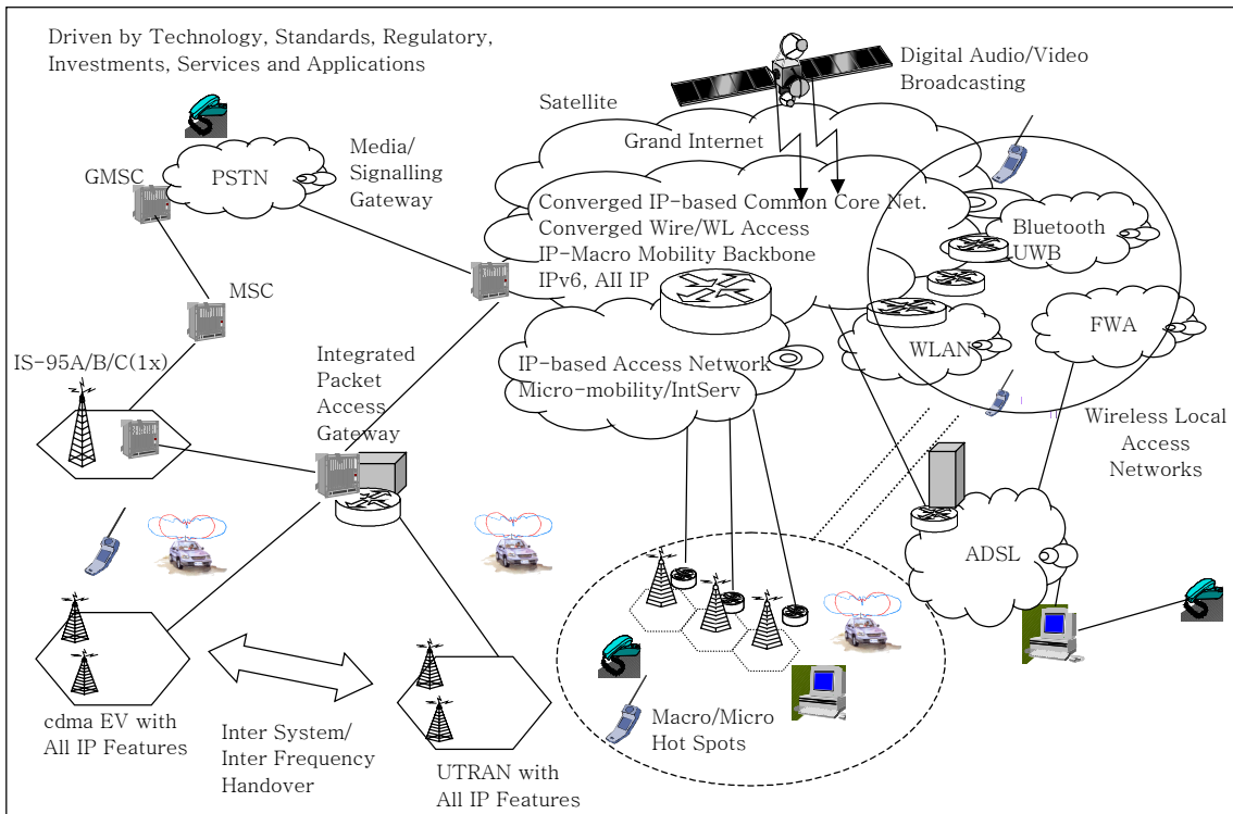
(그림 3) ETRI의 4G 무선전송기술 시스템 블록도
