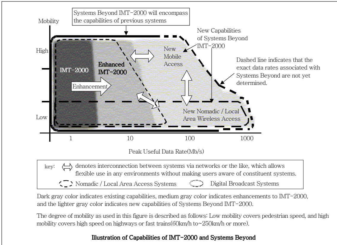
(그림 1) FDIMT와 SBIMT를 규정한 다이어그램
