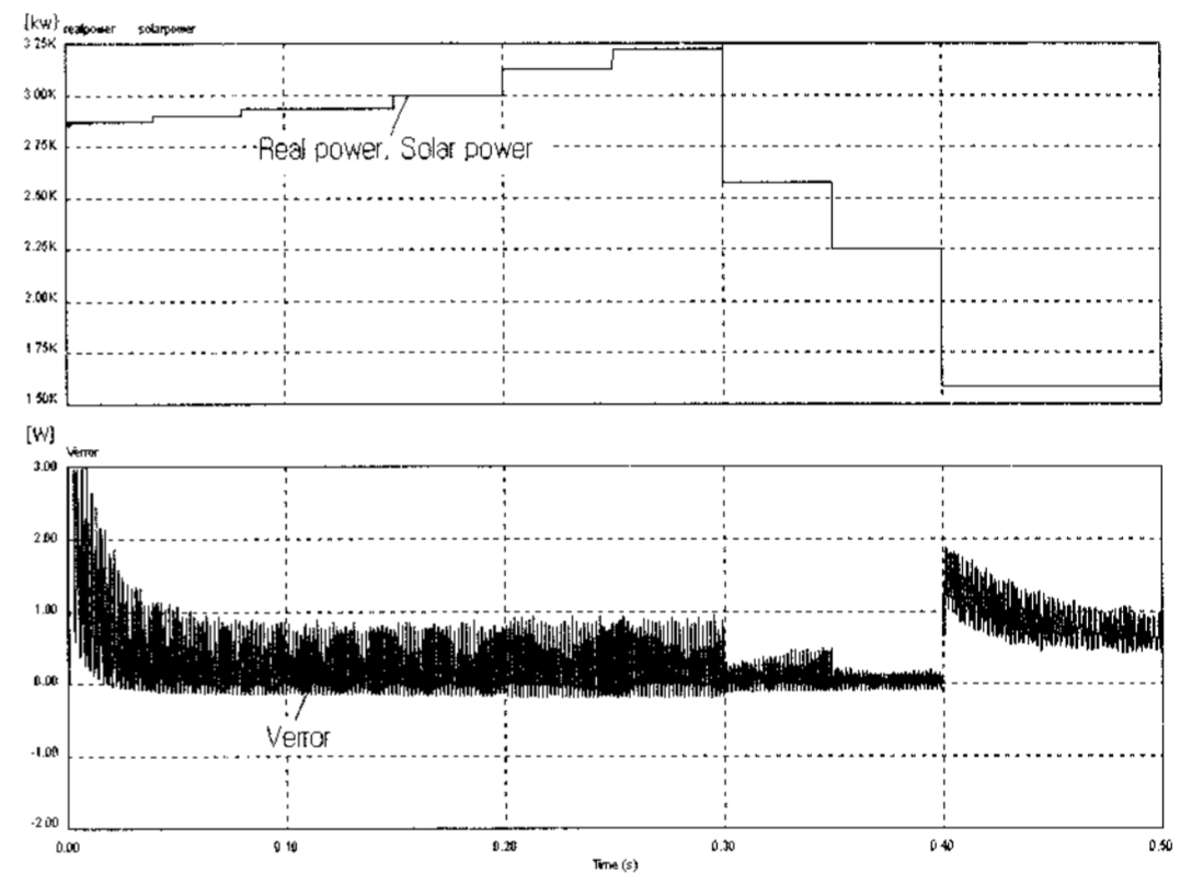
그림 11. Simulation results of IncCond MPPT
