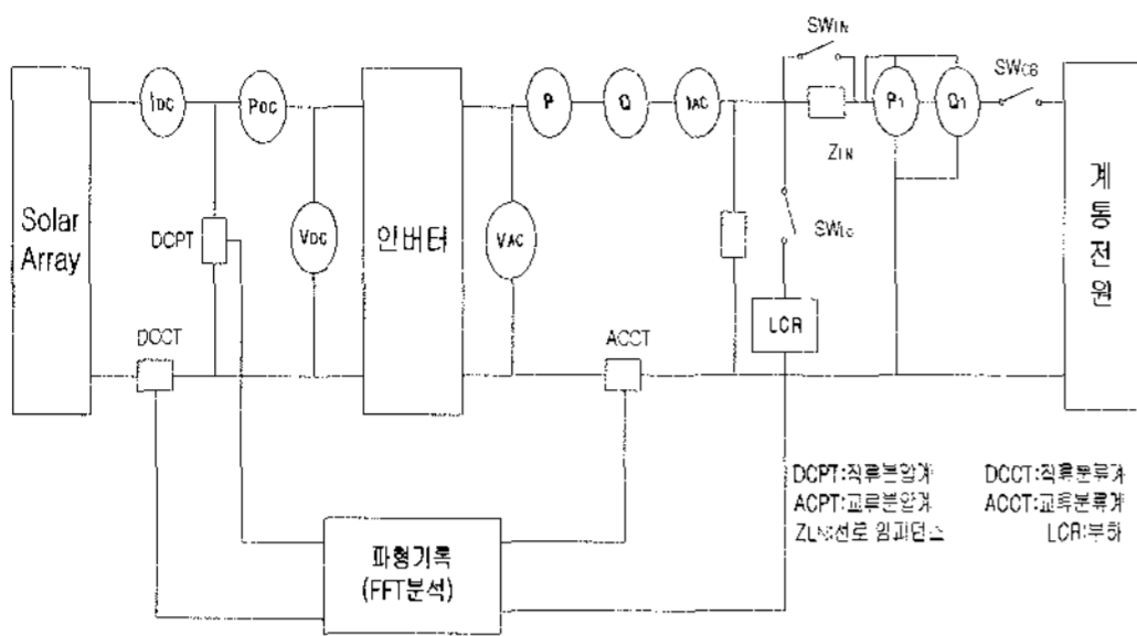
그림 7. Topology of MPPT efficiency measuring system
