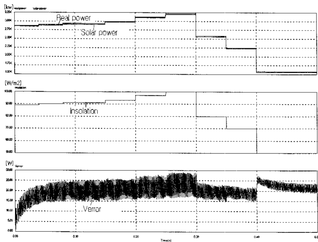
그림 9. Simulation results of constant voltage control MPPT
