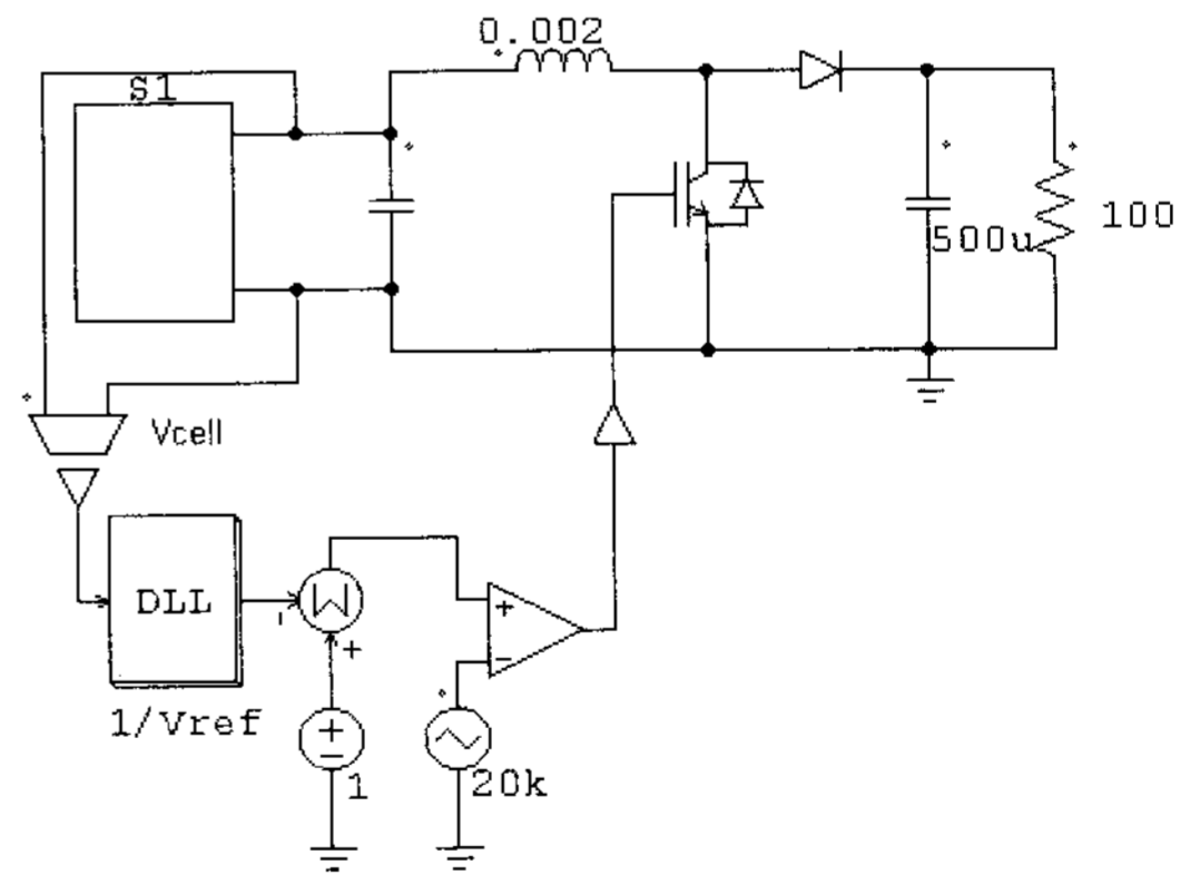
그림 3. Simulation of constant voltage control MPPT
