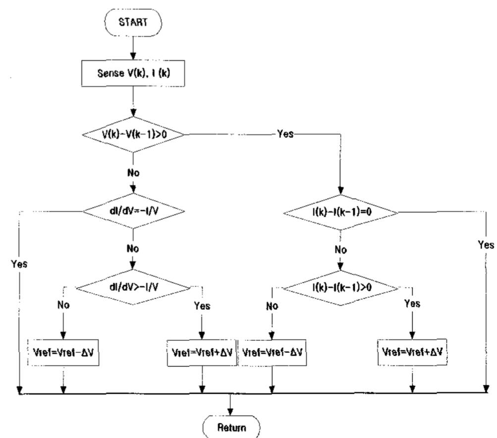
그림 5. IncCond MPPT algorithm flowchart
