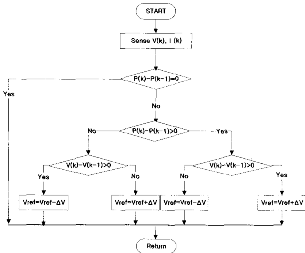
그림 4. P&O MPPT algorithm flowchart
