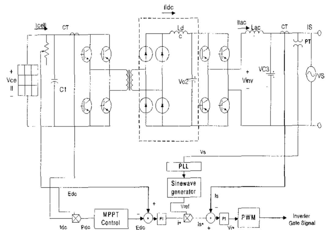
그림 8. Utility interactive inverter with high-frequency link
