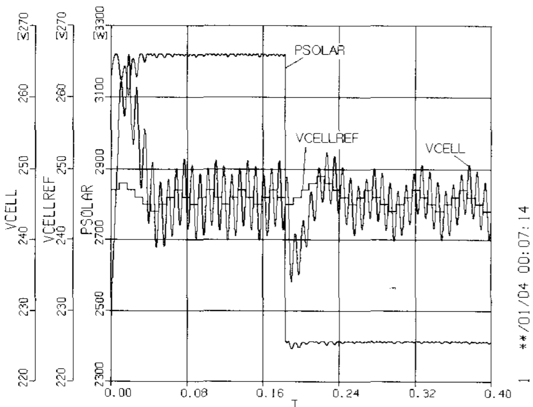
그림 14. Simulation results of P&O MPPT control in the utility interactive inverter
