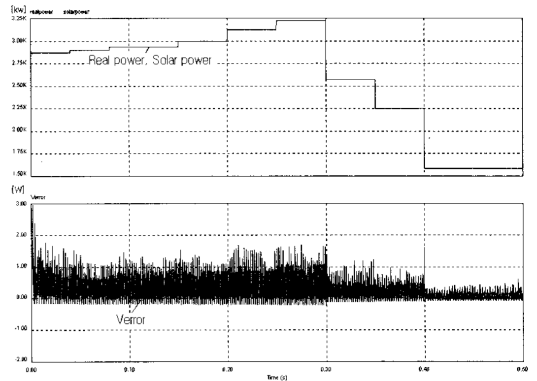
그림 10. Simulation results of P&O MPPT
