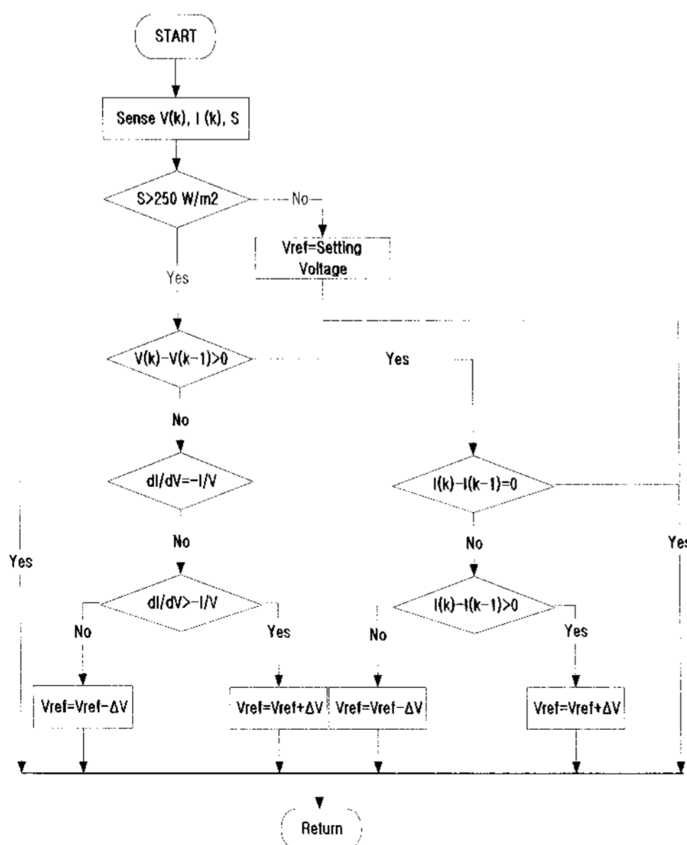
그림 6. Two-mode MPPT algorithm flowchart
