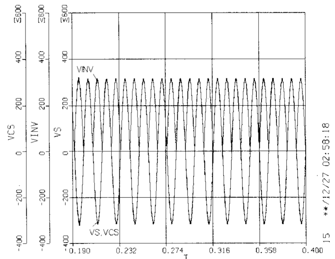
그림 12. Simulation results of utility interactive inverter
