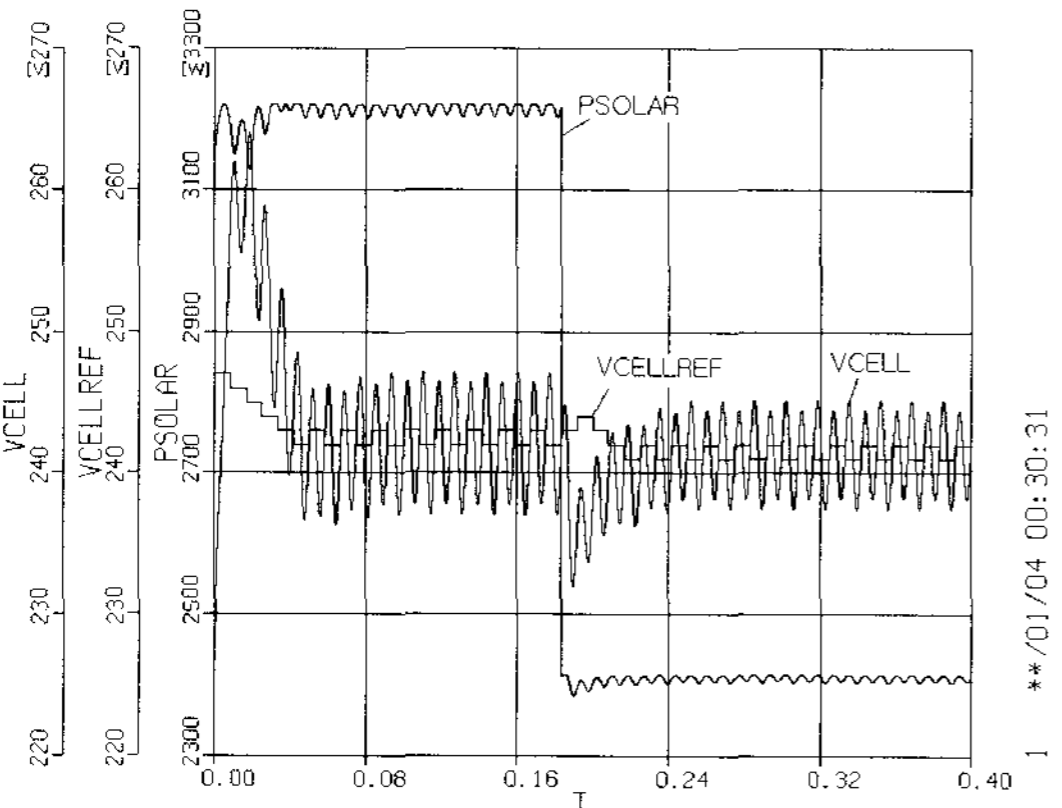
그림 15. Simulation results of IncCond MPPT control in the utility interactive inverter
