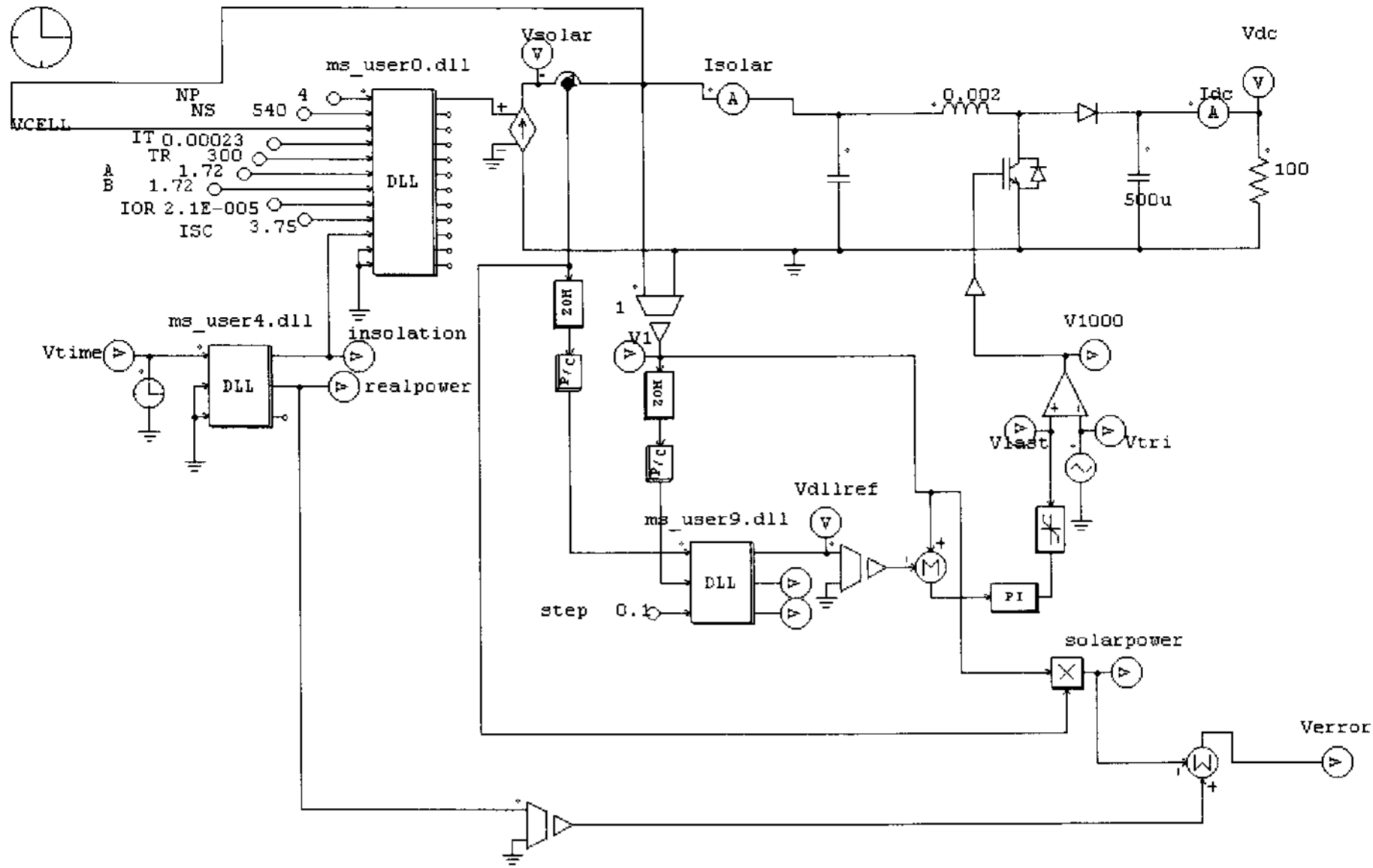
그림 2. Simulation circuit for MPPT performance
