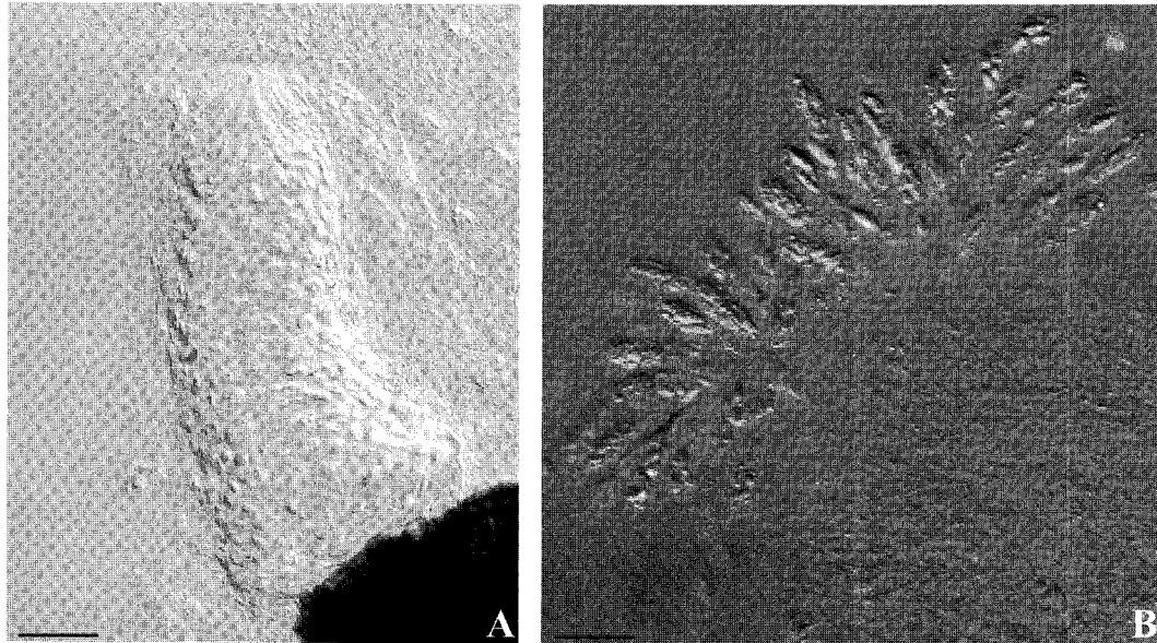
Fig. 2. Nitschkia confertula . A. Quellkörper. B. Asci. Scale bar : 25 \mu m.
