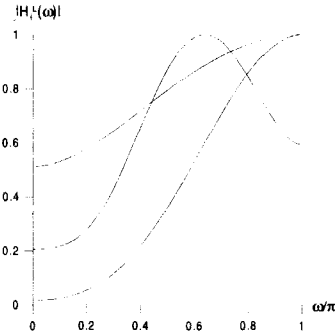
(a) 왼쪽 경계를 위한 경계필터의 주파수 특성
