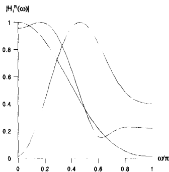
(b) 오른쪽 경계를 위한 경계필터의 주파수 특성
