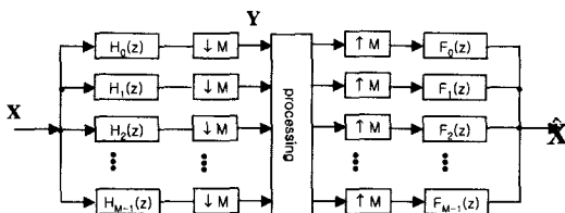
그림 1. M -대역 부대역 부호화기
