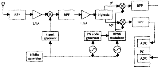
그림 7. 수신기 구성도
