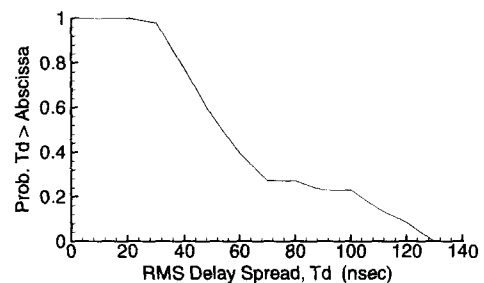
그림 13. 누적 RMS 지연분산
