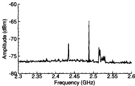
그림 15. 강남 도로변에서 2.4GHz 대역의 수신 잡음 특성
