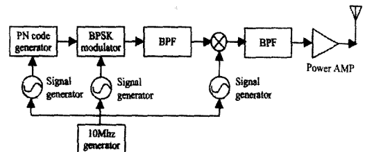
그림 6. 송신기 구성도
