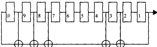
그림 2. PN 코드 발생기
