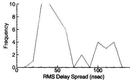
그림 12. RMS지연분산 히스토그램
