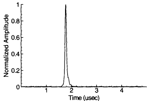
그림 10. 도심 10차선 도로의 10m 거리에서의 임펄스 채널 특성
