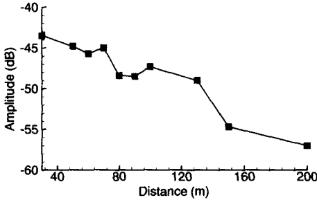
그림 14. 2.4GHz 대역에서의 거리에 따른 감쇠 특성
