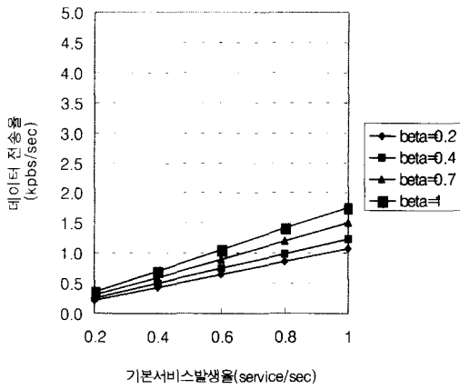
그림 2. 보안서비스를 위한 신호메세지 전송율 (평균 메시지 길이 : 256bits)
