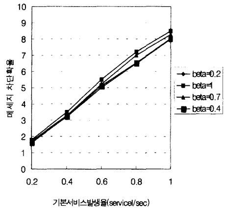
그림 5. 순방향 신호채널 메세지 차단확률 (신호채널 전송율 : 14.4kbps)
