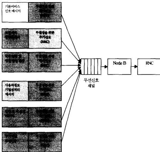
그림 1. 무선구간 신호채널 성능분석을 위한 채널 모델
