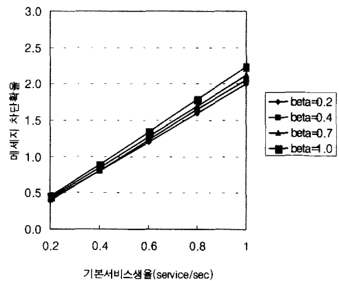
그림 7. 순방향 신호채널 메세지 차단확률 (신호채널 전송율 : 64kbps)
