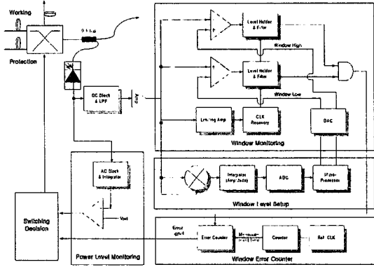
그림 3. 보호 절체 블록도
