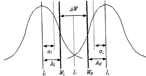
그림 2. 신호 분포와 윈도우 레벨의 관계
