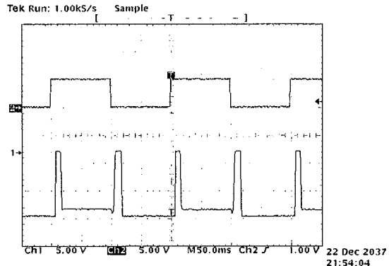
채널 위:스위칭 펄스 채널아래:수신 광세기(신호존재시 LOW)
