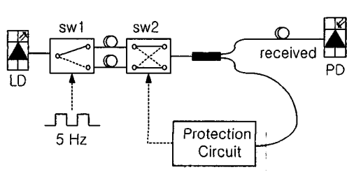
그림 4. 선로 사고 모의 실험
