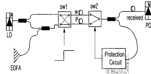
그림 6. ASE잡음으로 인한 성능 저하 모의 실험
