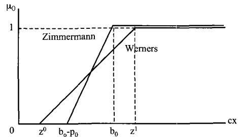
그림 6. Zimmermann과 Werners의 멤버십함수
