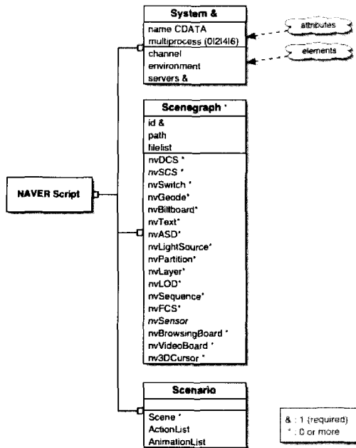
그림 3. NAVER 스크립트의 구조
