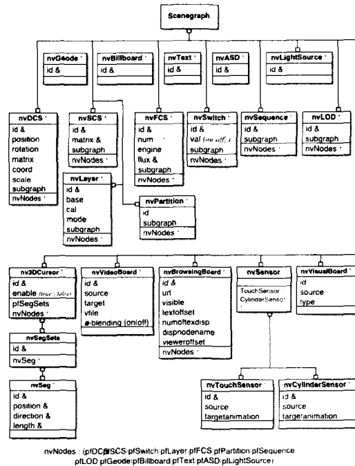
그림 5. NAVER 스크립트의 Scenegraph 정의 부분
