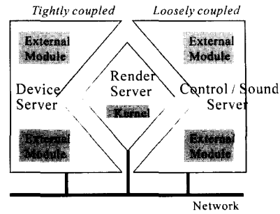
그림 1. NAVER의 기능적 구성
