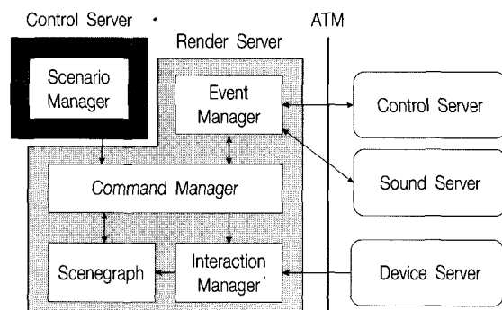
그림 2. NAVER 커널과 외부 서버와의 연결
