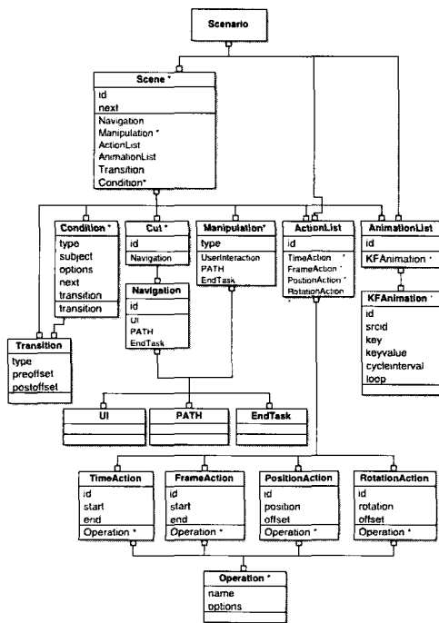
그림 6. NAVER 스크립트의 Scenario 정의 부분
