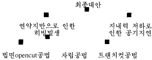
그림 5. 흙막이 및 터파기 공종의 계층분류체계
