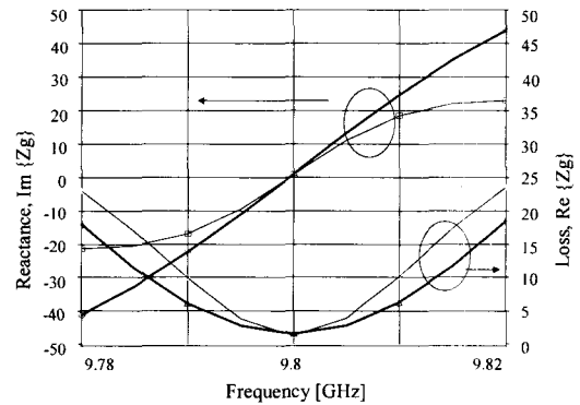
그림 4. 공진주파수 근처에서 Zg의 궤적
