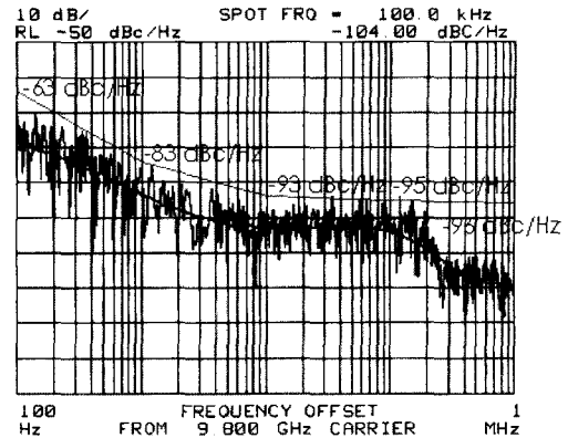
그림 10. 위상잡음 특성 Fig. 10. Phase noise characteristics.
