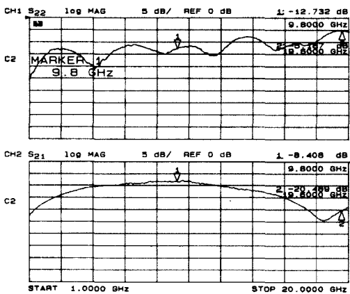
그림 8. 방향성 결합기의 반사계수 및 결합 특성
