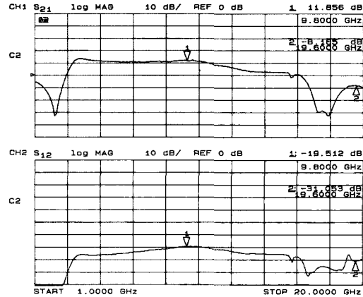
그림 6. 완충증폭기의 이득 및 분리도 특성
