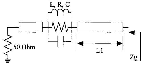
그림 3. 마이크로스트립라인과 결합한 유전체 공진기의 등가회로
