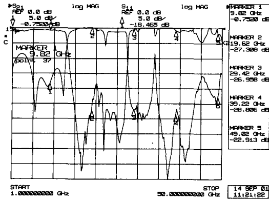
그림 7. 저역통과필터의 삽입손실 및 고조파 억압 특성
