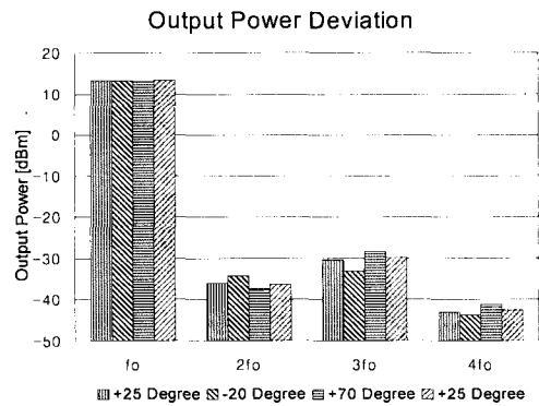
그림 12. 온도변화에 대한 출력변화 특성 Fig. 12. Output power deviation for temperature variation.
