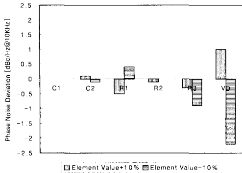
그림 5. 집중소자 및 바이어스 변화에 따른 위상잡음의 변화
