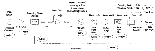
그림 1. 국부 발진기의 구성도
