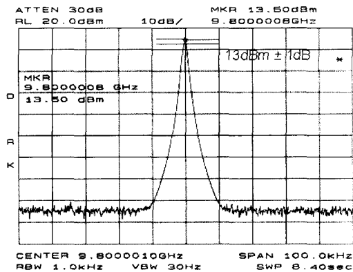
그림 9. 출력전력 특성 Fig. 9. Output power characteristics.
