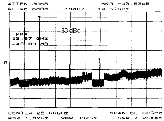
그림 11. 고조파 억압특성 Fig. 11. Harmonic suppression characteristics.
