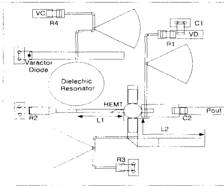
그림 2. 전압제어 발진기의 구조 Fig. 2. The structure of VCO.
