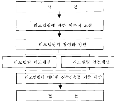
그림 1. 연구의 흐름도
