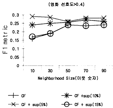
<그림 3> 선호도 0.4 이상인 영화에 대해 협력적 여과 방식과 연관 규칙을 같이 사용한 협력적 여과 방식과의 비교
