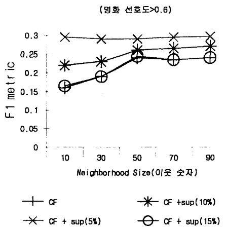
<그림 4> 선호도 0.6 이상인 영화에 대해 협력적 여과 방식과 연관 규칙을 같이 사용한 협력적 여과 방식과의 비교
