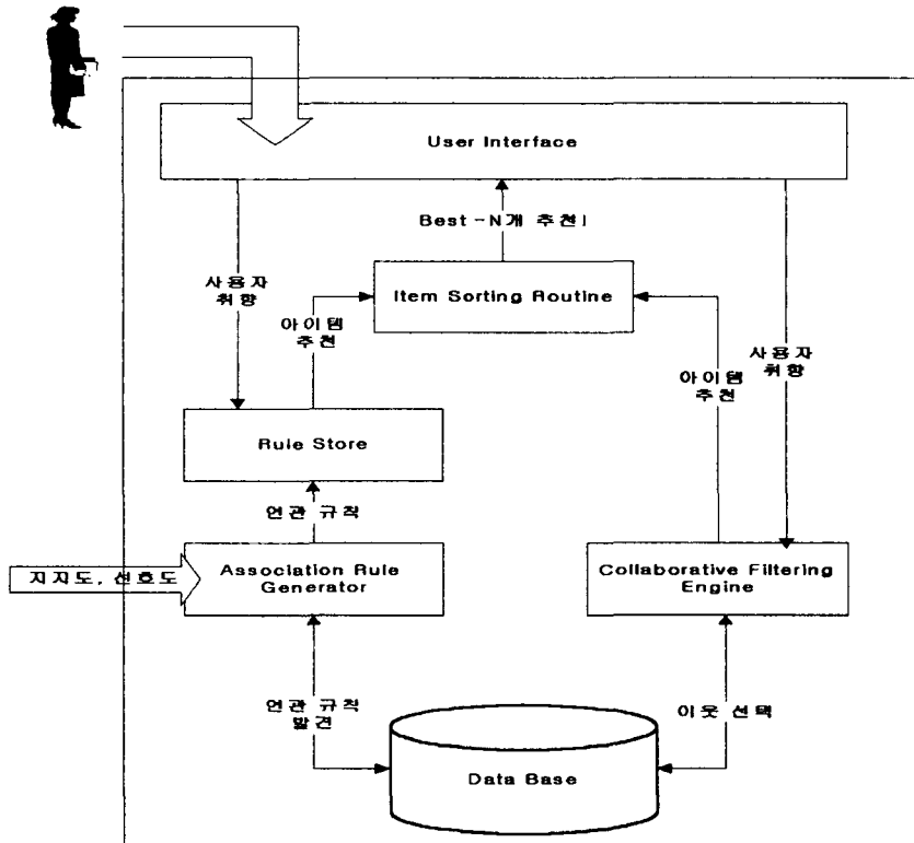
<그림 1> 추천 시스템의 전체 구조
