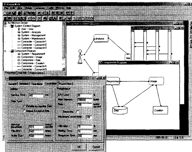
<그림 2> HappyWork 환경
