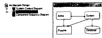
<그림 5> Component Diagram
