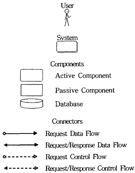
<그림 3> 아키텍처 구성 요소
