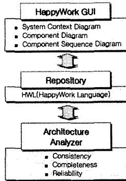
<그림 1> HappyWork 구조
