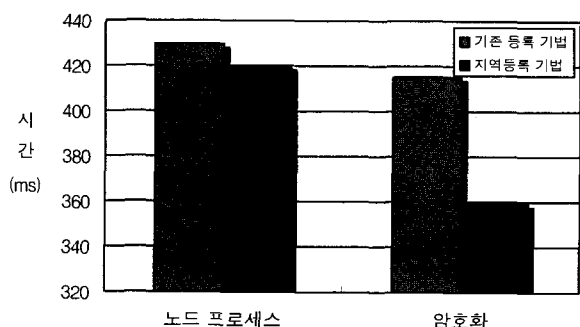
(그림 20) 노드 프로세스 시간, 암호화 시간(최소 공개키 메커니즘)
