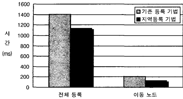
(그림 14) 전체 등록 시간 비교(공개키 메커니즘)
