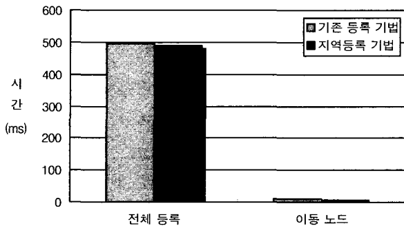
(그림 15) 전체 등록 시간 비교(최소 공개키 메커니즘)
