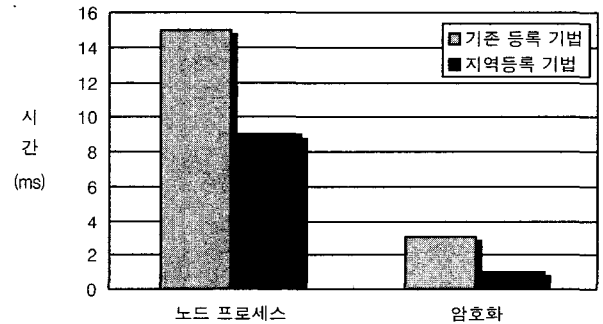
(그림 18) 노드프로세스 시간과 암호화 시간(비밀키 메커니즘)
