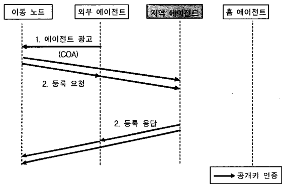
(그림 8) 지역 등록시 공개키 기반 인증 메커니즘 동작
