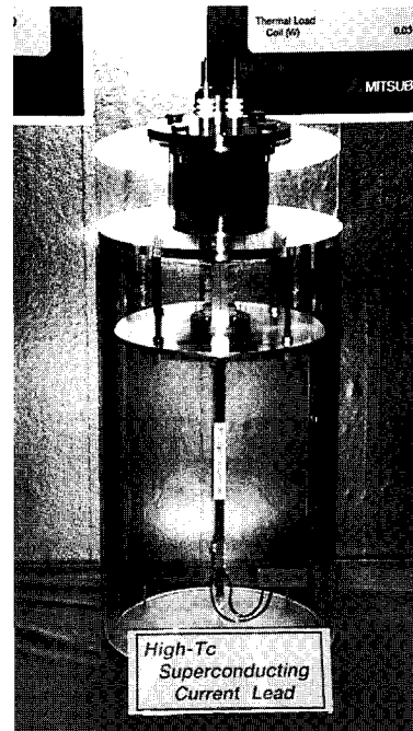
그림 6. 용융-주조공정으로 제조한 벌크형 BSCCO 전류인입선 (ACCEL Intr. Co.)과 BSCCO 테이프형 초전도체(일본)
