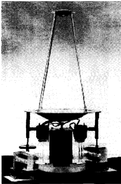
그림 8. NASA에서 개발한 초전도 베어링을 사용한 천체 망원경
