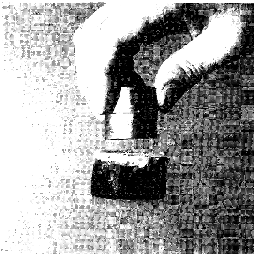
그림 3. 영구자석 밑에 매달린 YBCO 초전도체
