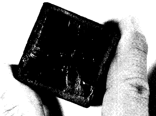
그림 1. 종자결정 성장법으로 제조한 일방향 성장 YBCO 초전도체
