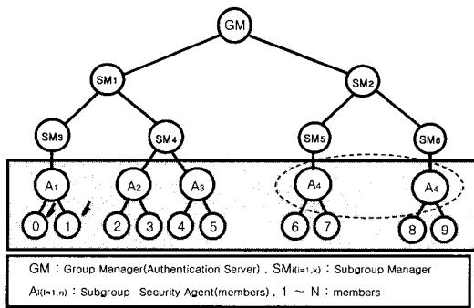
(그림 3) 키 그룹 트리
