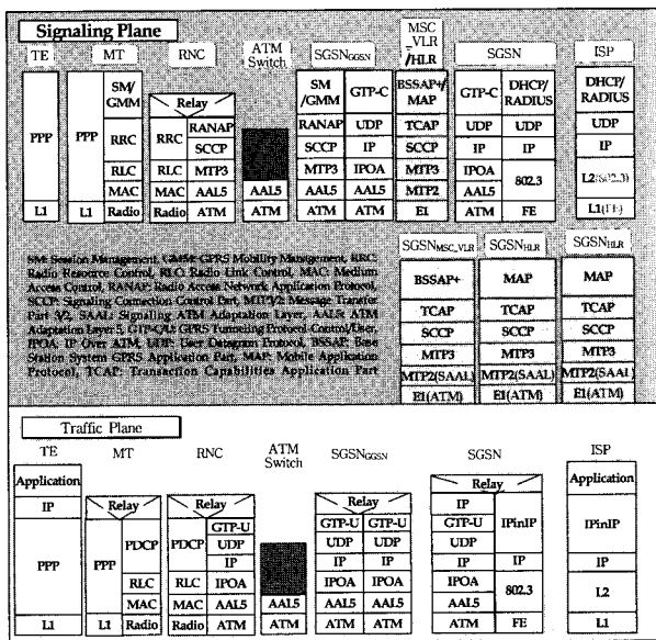
(그림 3) 이동 ISP 가입자가 GPRS 망을 통해 홈 ISP 망 접속시 신호 및 데이터 처리에 필요한 프로토콜 스택 구조
