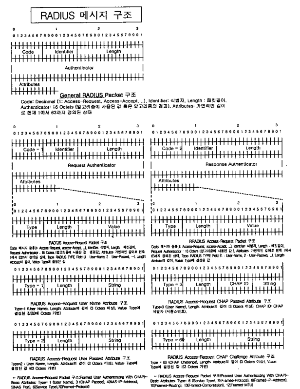
(그림 8) RADIUS Client 메시지 구조
