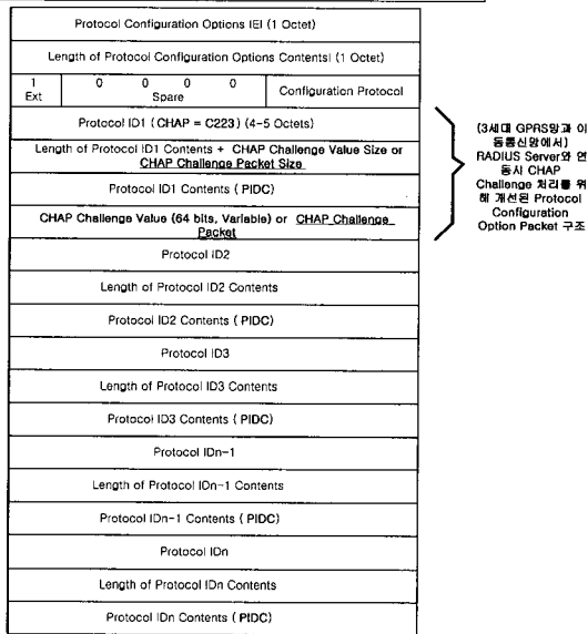
(그림 6) MT PCO 구조에서 PPP CHAP Challenge 값의 처리 구조 정의
