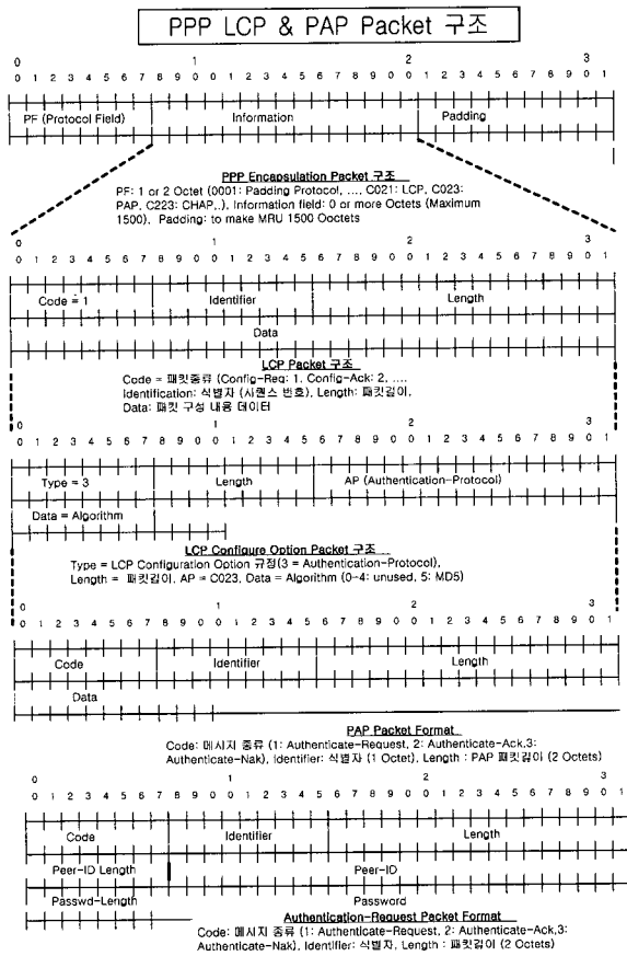
(그림 1) PPP LCP & PAP 메시지 구조
