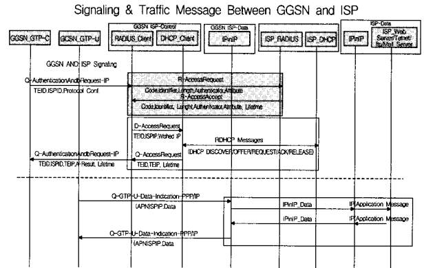
(그림 7) GPRS GGSN과 ISP RADIUS/DHCP 사이의 인터워킹 메시지
