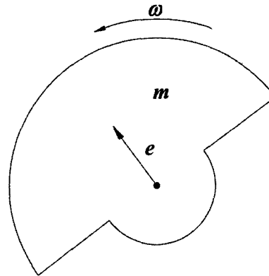
Fig. 2 Eccentric rotor
