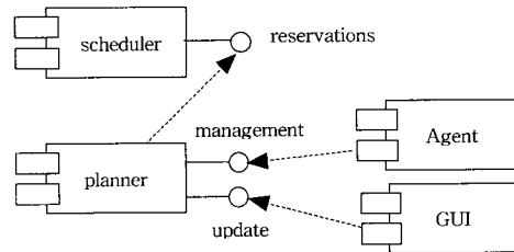
(그림 12) UML 컴포넌트 다이어그램
