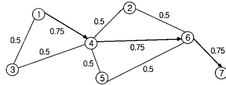
(그림 2) 식 (2)를 적용한 후 네트워크 예제 ( l_1(e) )
