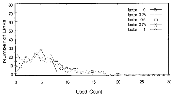
(그림 4) 부하균등의 시뮬레이션 결과(300개의 연결)
