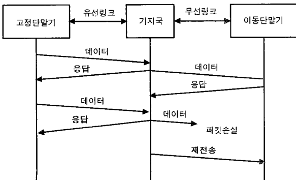
(그림 2) I-TCP의 동작원리
