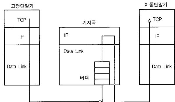
(그림 3) Snoop 모듈의 동작원리
