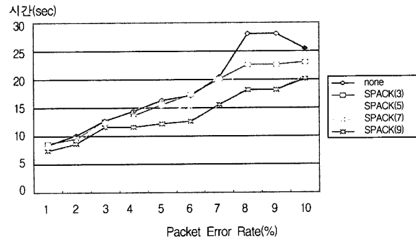
(그림 9) 패킷손실율 vs. 전송시간(MSS = 500B)
