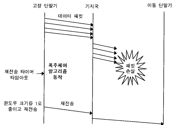
(그림 1) 무선통신 환경에서 TCP의 동작
