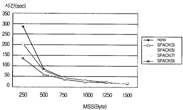
(그림 13) MSS vs. 전송시간(500KB전송)
