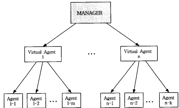
(그림 14) 확장성을 고려한 관리 모델
