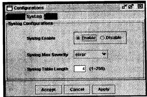
(그림 13) 시스템 로그의 설정
