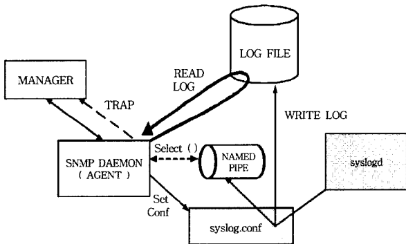
(그림 6) CNU-SYSLOG-MIB의 동작
