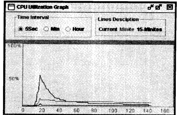
(그림 9) 연속적인 정보요청을 통한 성능 감시
