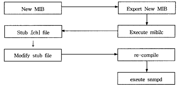
(그림 4) MIB 및 모듈 추가 절차
