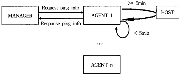
(그림 5) CNU-PING-MIB의 동작
