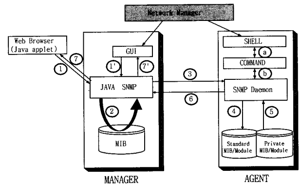
(그림 2) 매니저-에이전트간 EMS 동작과정
