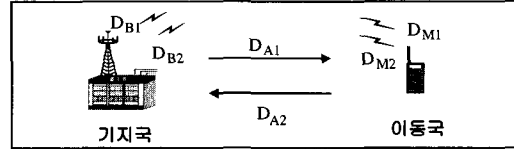
그림 3. RTD 모델
