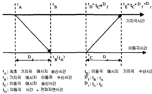
그림 2. 메시지 처리과정
