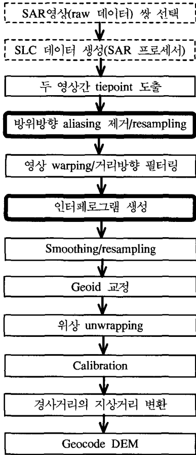
그림 1. IFSAR 알고리즘
