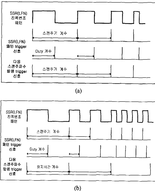
그림 8. SSR 패턴 발생 알고리즘 (a) 유지시간이 없는 경우 (b) 유지시간이 있는 경우
