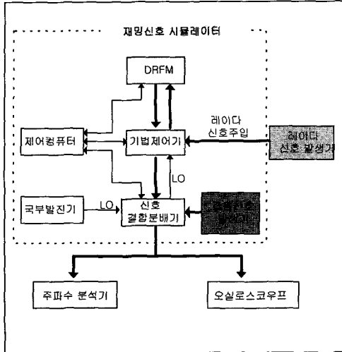
그림 10. 시험장비 구성
