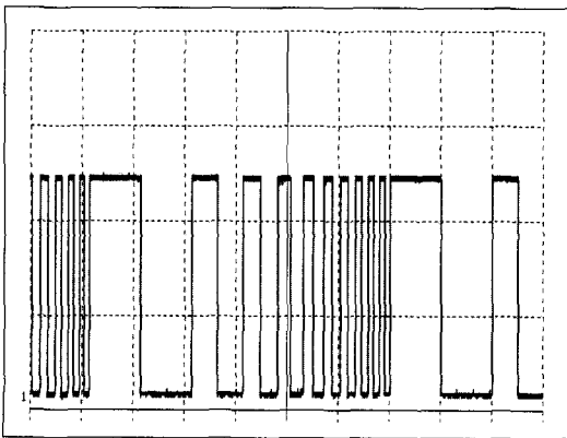
그림 21. 유지시간이 없는 SSR 발생결과
