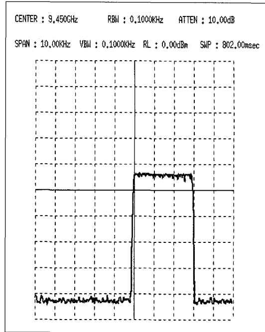
그림 17. 2.9kHz 주파수 편향 VGPO 발생결과
