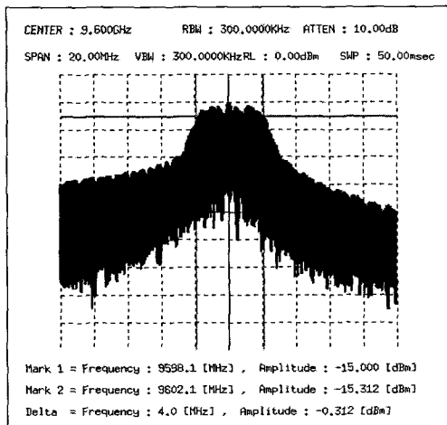
그림 11. 점잡음 발생결과(잡음대역폭=4MHz)
