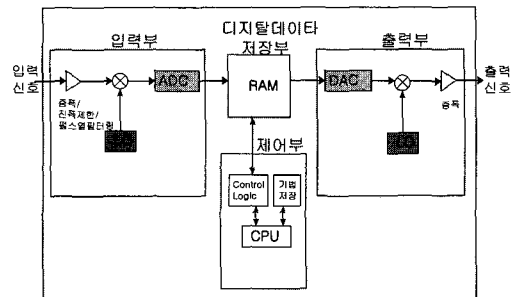
그림 2. DRFM 구성도
