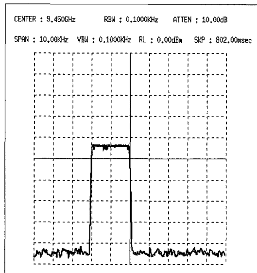
그림 18. -1.9kHz 주파수 편향 VGPI 발생결과
