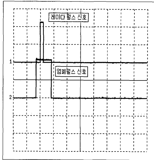
(a) 엄폐 펄스 발생결과(펄스 폭=20 \mu s)
