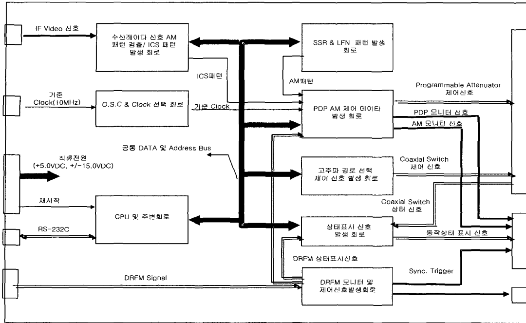
그림 5. 기법제어기 제어회로 계통도
