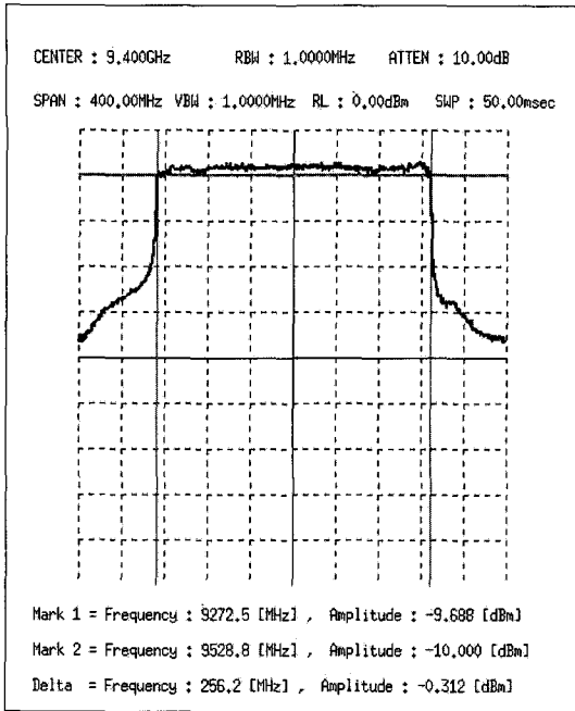
(b) 소인대역폭(=256MHz)
