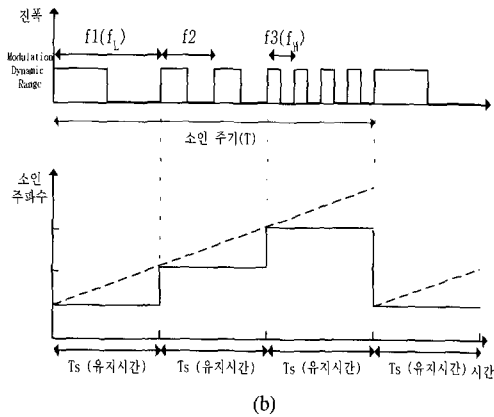
그림 7. SSR 기법 발생 형태 (a) 비선형 소인 형태 (b) 선형 소인 형태
