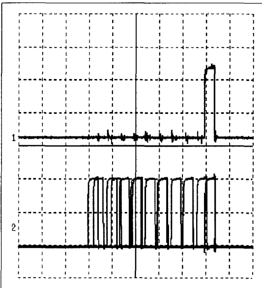
그림 16. 75 % 속력의 RGPI 발생결과
