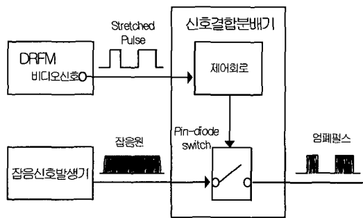
그림 3. 엠펜펄스 구현 방법
