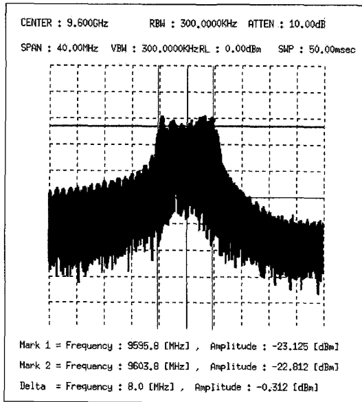
(b) 잡음신호 발생결과(잡음 대역폭=8MHz)
