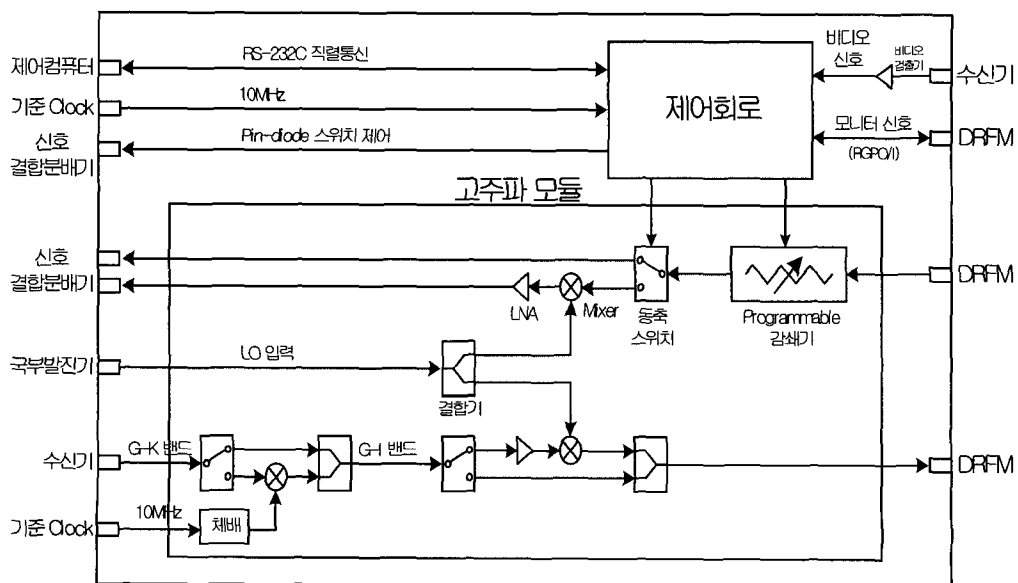
그림 4. 기법제어기 계통도
