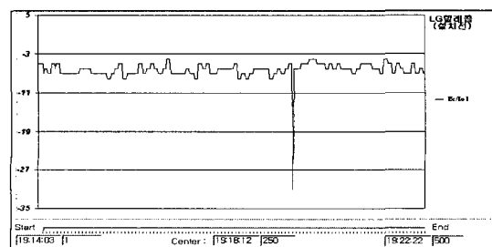
그림 13. LG 텔레콤 단말기의 Ec/Io(설치 전)
