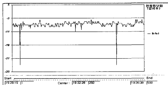
그림 10. 한통엠닷컴 단말기의 Ec/Io(설치 후)
