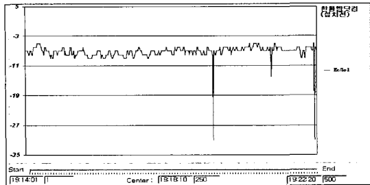
그림 9. 한통엠닷컴 단말기의 Ec/Io(설치 전)
