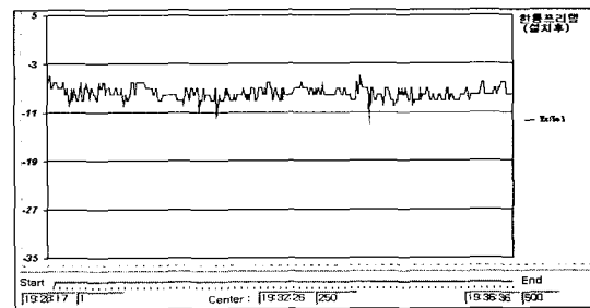
그림 6. 한통프리텔 단말기의 Ec/Io(설치 후)
