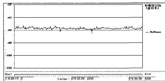
그림 12. 한통엠닷컴 단말기 수신전력(설치 후)
