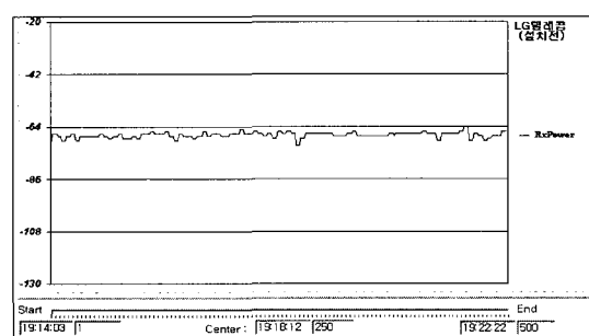
그림 15. LG 텔레콤 단말기 수신전력(설치 전)
