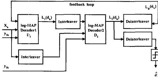
그림 2. log-MAP 터보복호기
