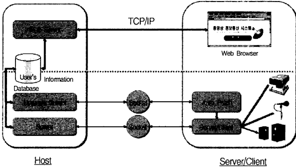
(그림 6) 화상 진료 시스템의 구성
