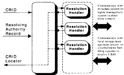
그림 5 CRID Resolution Architecture
