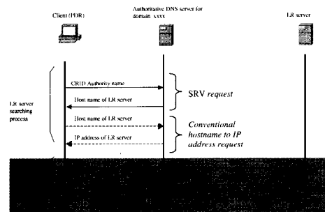
그림 6 TCP/IP를 이용한 CRID Resolution
