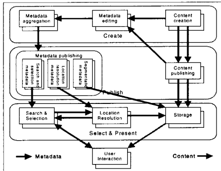
그림 4 Metadata와 콘텐츠 흐름
