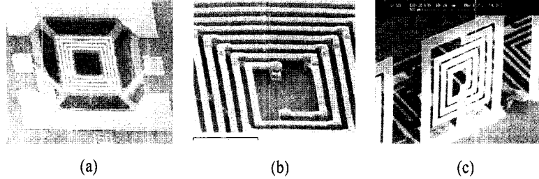
[그림 8] RF MEMS 3-D spiral type 인덕터
