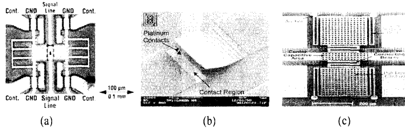
[그림 3] RF MEMS 저항형 스위치
