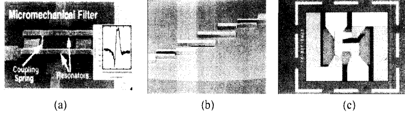
[그림 10] RF MEMS 필터
