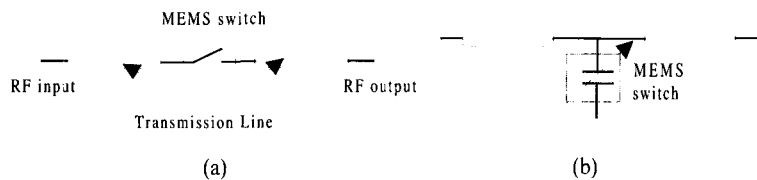
[그림 2] RF MEMS 스위치의 개념도: (a) 저항형 스위치, (b) 용량형 스위치
