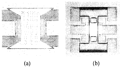
[그림 4] RF MEMS 용량형 스위치
