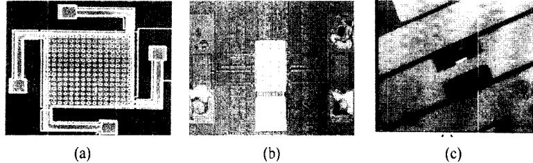
[그림 5] RF MEMS 가변 커패시터
