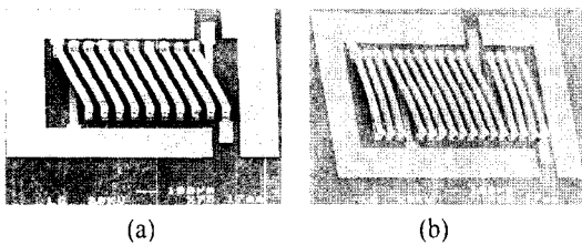
[그림 9] RF MEMS 3-D solenoid type 마이크로 트랜스포머
