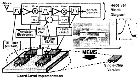
[그림 1] RF 송수신기에 RF MEMS기술의 적용 예
