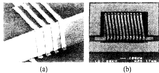
[그림 7] RF MEMS 3-D solenoid type 인덕터 (a) alumina core를 이용한 인덕터(버클리대학) (b) 기판위에 띄운 air core 인덕터(LG)
