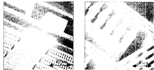
[그림 6] RF MEMS 가변 커패시터: 정전력 구동의 interdigitized comb 구조(Rockwell)
