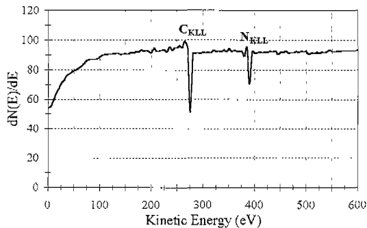
그림 1. 자장의 도움이 없이 0.1 Torr, 4.0 kV에서 증착한 두께가 1.4 \mu m인 질화탄소 시료의 Auger 전자 스펙트럼.
