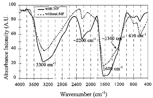
그림 4. 0.1 Torr와 4.0 kV의 조건에서 증착한 질화 탄소 박막의 IR 스펙트럼 : (실선) 자장의 도움 유; (점선) 자장의 도움 무.
