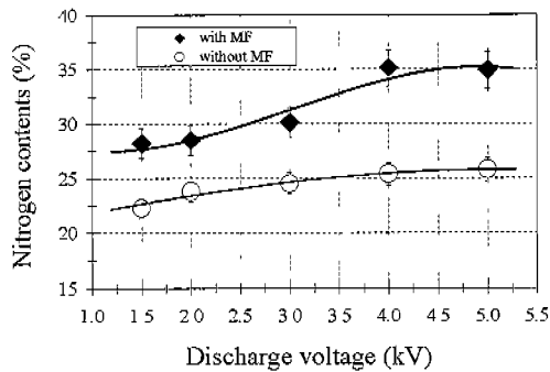
그림 2. 0.1 Torr에서 증착한 시료들의 방전 전압(kV)에 따른 질소 함유량 변화.
