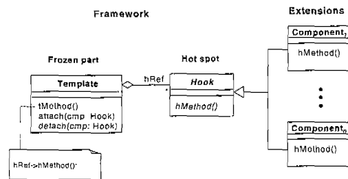
그림 5 Hot Spots of a framework
