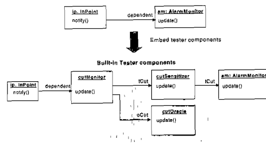
그림 16 Embedding BIT in an AlarmMonitor
