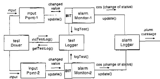
그림 17 A Possible Object Structure of BIT-Embedded Alarm Monitoring System
