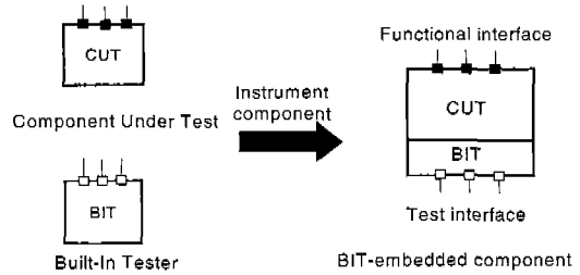
그림 1 Embedding BIT in CUT
