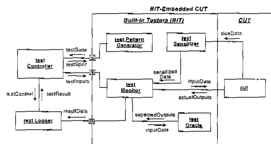
그림 3 BIT-Embedded CUT
