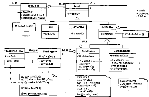
그림 6 Class Structure of BIT-Embedded Framework Hot Spot
