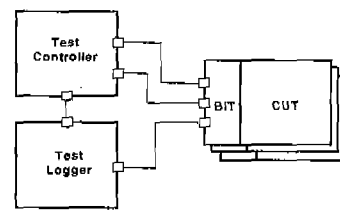
그림 4 BIT-Embedded FUT
