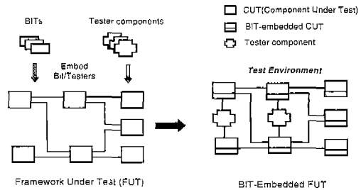
그림 2 Embedding BIT's in a FUT
