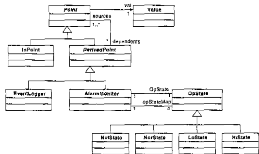
그림 10 Partial Class Structure of the Alarm Monitoring Framework
