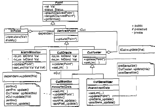
그림 15 Class Structure of BIT-Embedded Alarm Monitor
