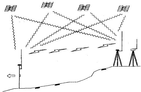
그림 4. RTK GPS 측위방법의 구성
