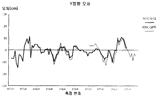
그림 10. Y방향 오차
