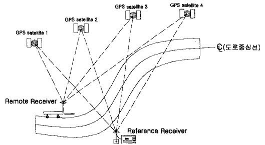
그림 6. 관측시스템의 구성
