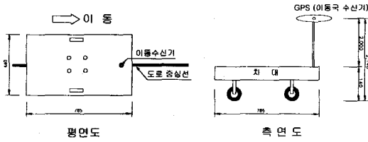
그림 7. 관측시스템 중 차대의 구성
