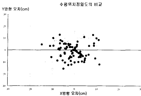
그림 11. 수평위치정밀도의 비교
