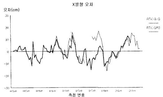
그림 9. X방향 오차
