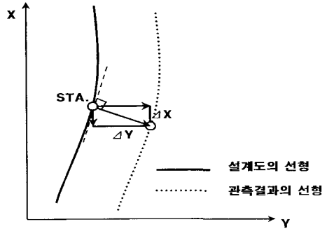
그림 8. 비교방법
