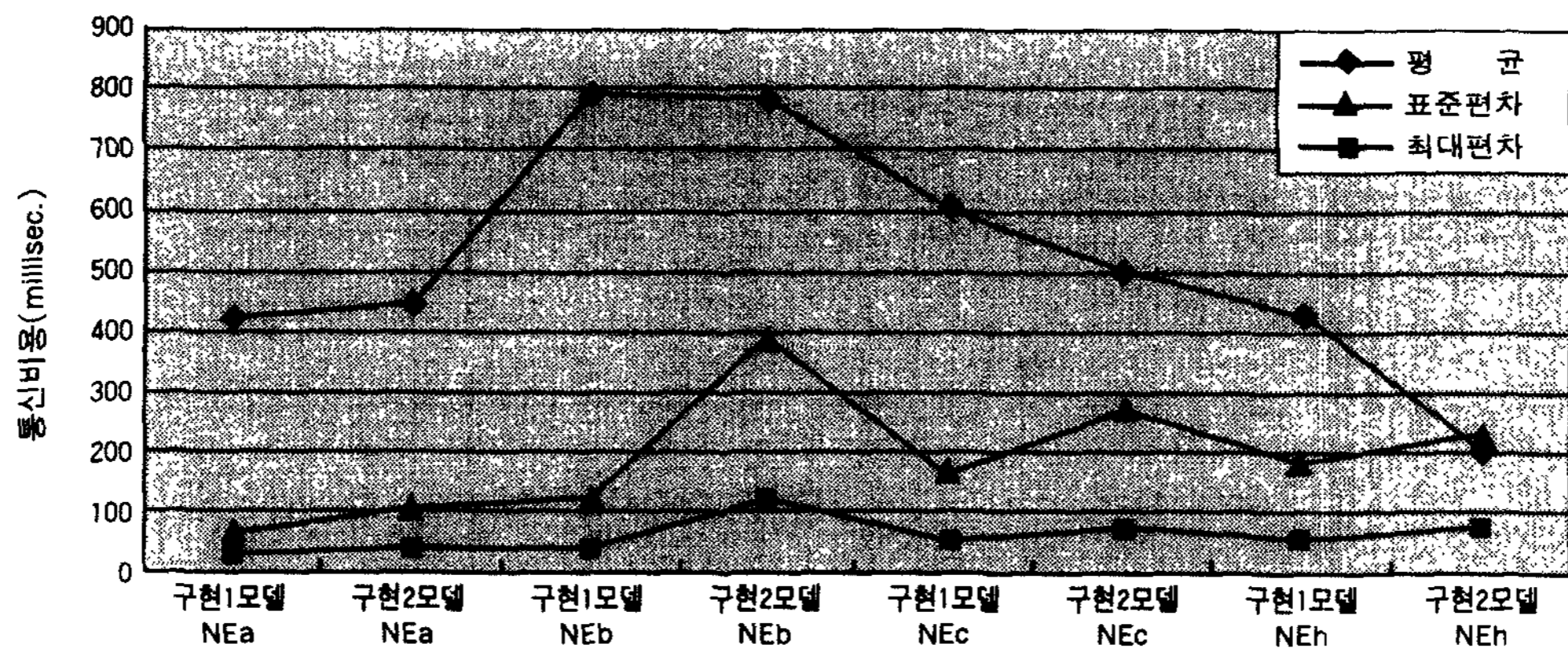
〈그림 17〉 두 모델의 통신비용에 대한 평균과 표준 편차, 최대 편차
