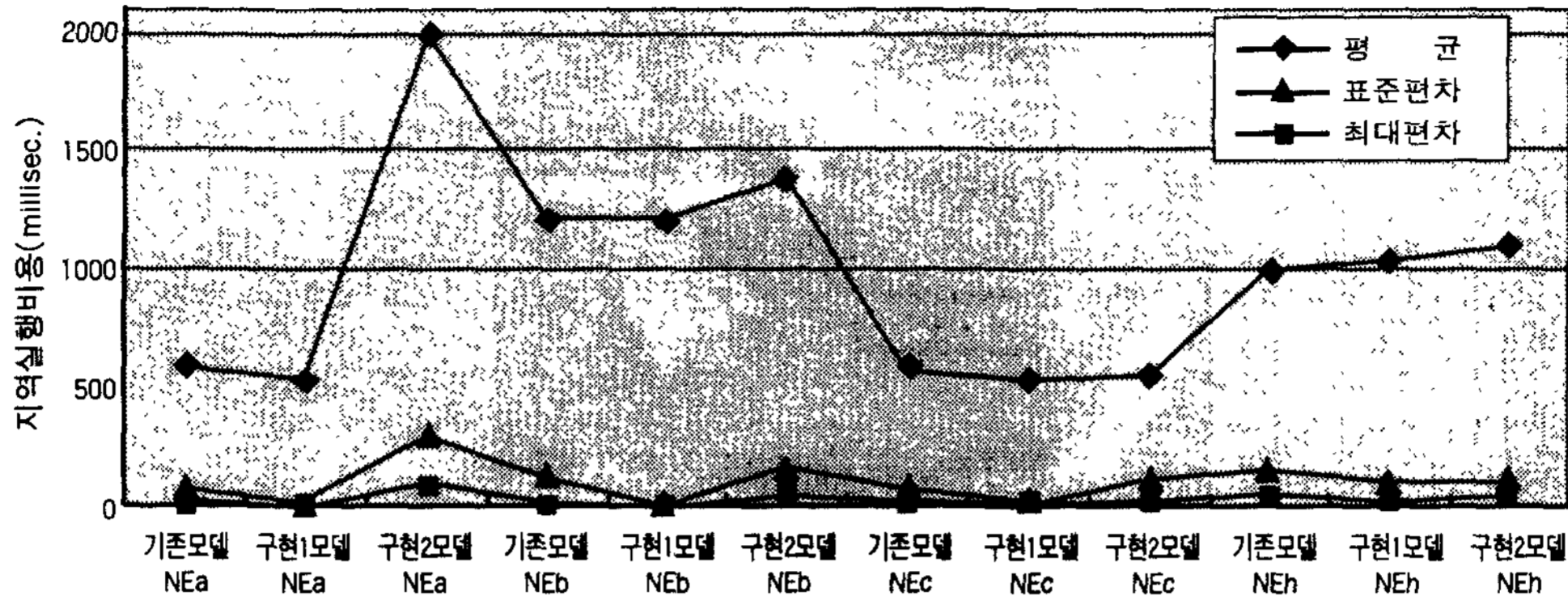
〈그림 16〉 각 모델별 지역 실행비용의 평균과 표준 편차, 최대 편차
