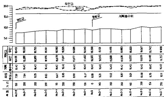
그림 4. 대상지역의 종단면도
