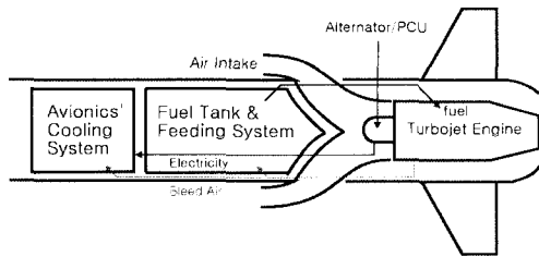
Fig. 206 전형적인 추진기관 시스템의 구성
