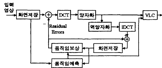
(a) MPEG-2 비디오 인코더
