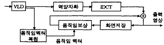
(b) MPEG-2 비디오 디코더
