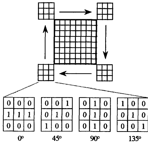
〈그림 5〉 방향성 검출부
