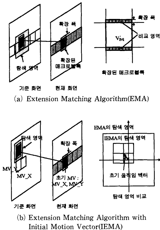
〈그림 7〉 확장 영역을 이용한 움직임 벡터 추정
