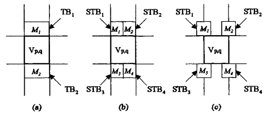
〈그림 6〉 이웃 매크로블록의 움직임 벡터의 평균
