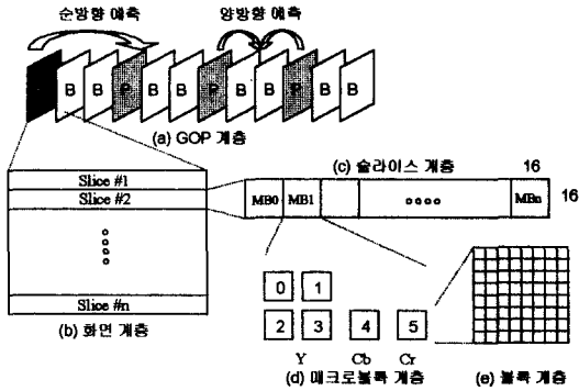
〈그림 2〉 MPEG 영상의 계층적 구조
